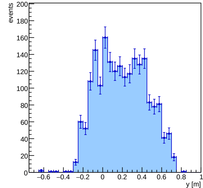
Vertex y
