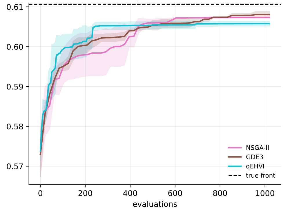
ImageNet16-120
