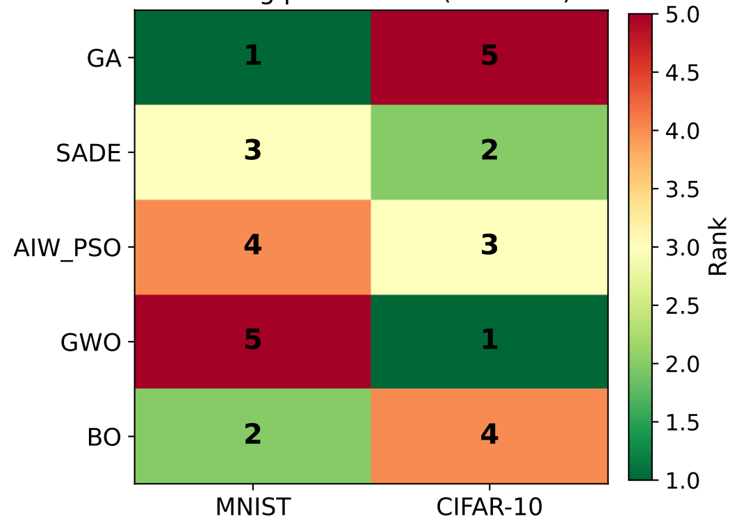
Ranking per dataset (1 = best)
