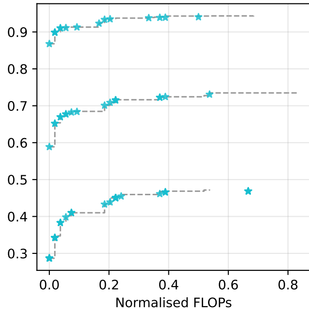
qEHVI
