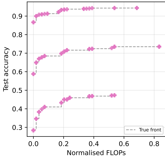
NSGA-II
