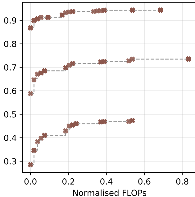
GDE3
