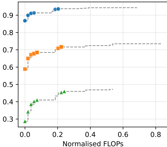
SADE
