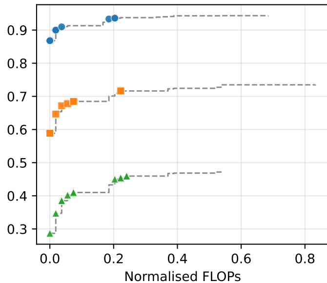
BO
