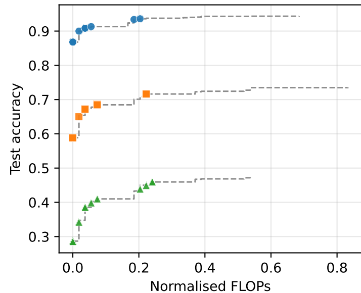
GWO
