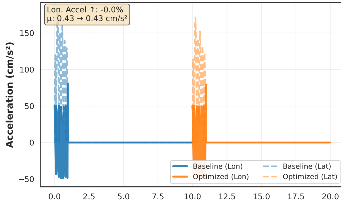
A) Longitudinal & Lateral Acceleration
