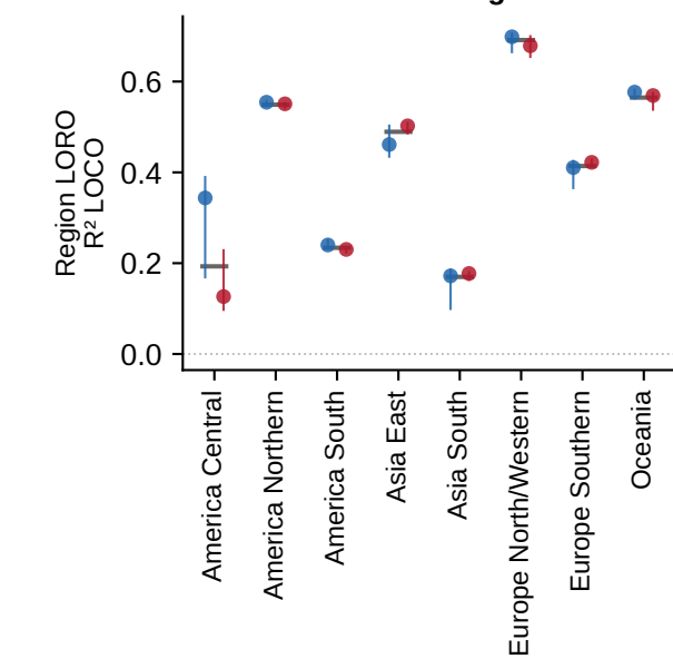
d. Functional BAG Region LORO
