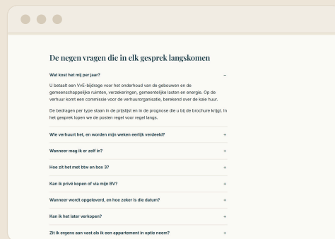
De vragen uit elk gesprek, vooraf beantwoord
