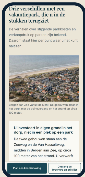
Drie verschillen met een vakantiepark
