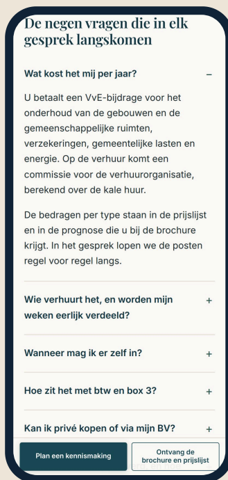
De vragen uit elk gesprek
