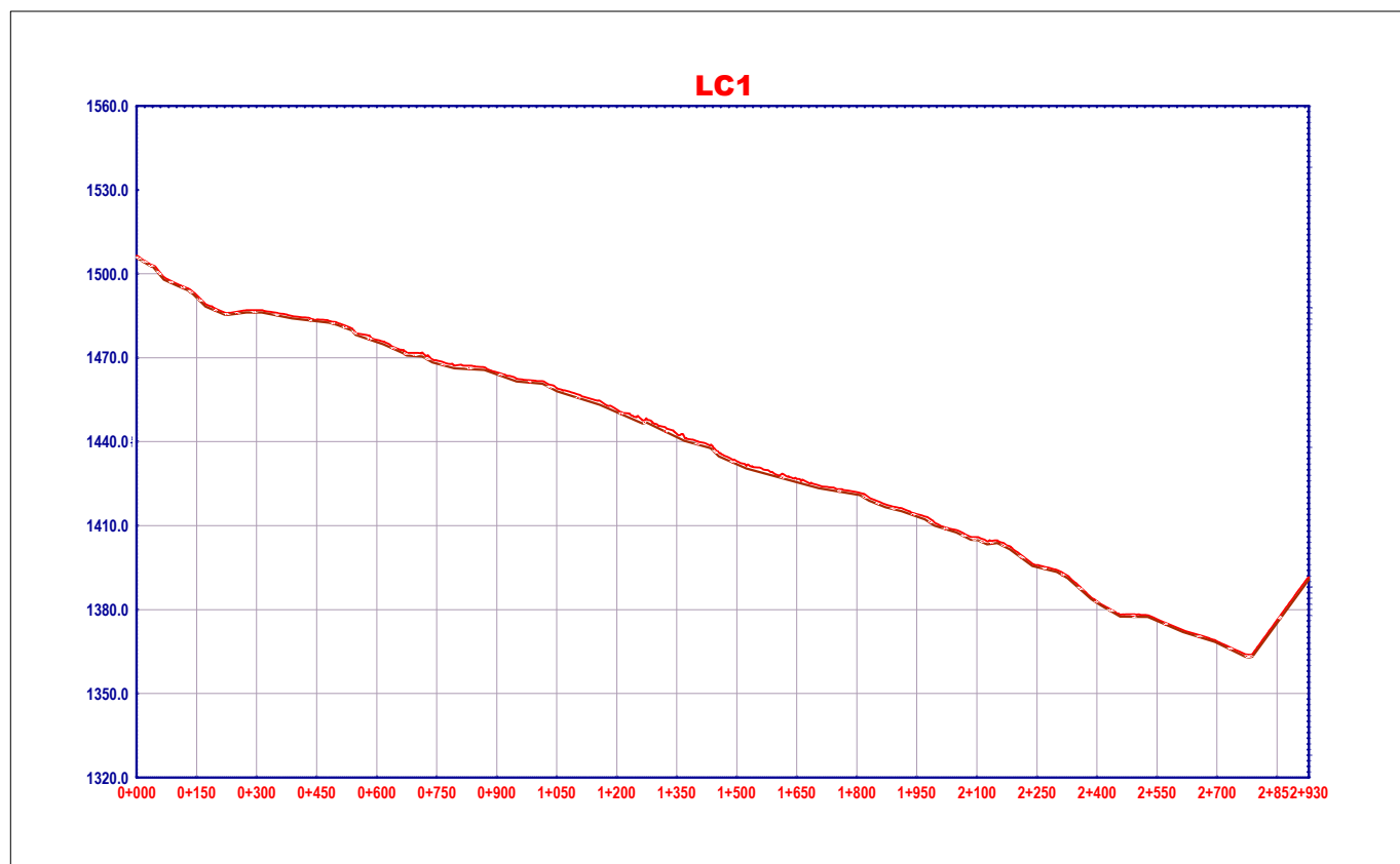
PERFIL LONGITUDINAL HORIZ.=1:1000 VER.=1:100
