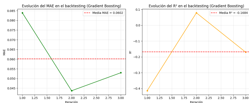
Figura 4.5: Graficas de la evolución de MAE y R 2 a lo largo de las iteraciones del backtesting. Fuente de elaboración propia
