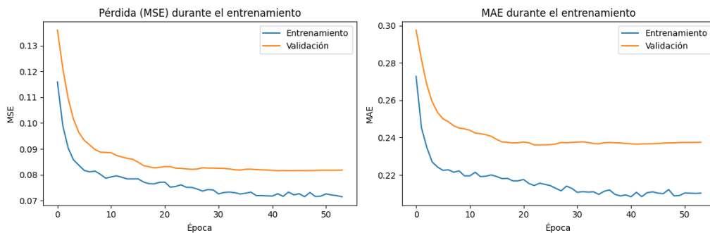
Figura 4.1: Evolución de la pérdida (MSE) y del MAE durante el entrenamiento de la LSTM.
