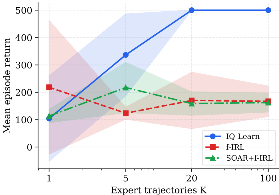
CartPole-v1 (best return)
