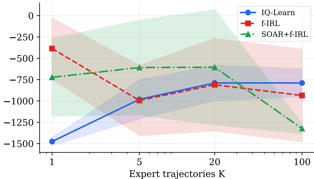
Pendulum-v1 (best return)
