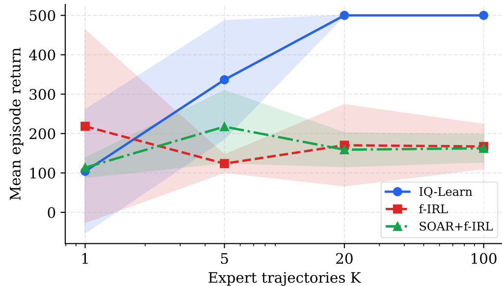
CartPole-v1 (best return)
