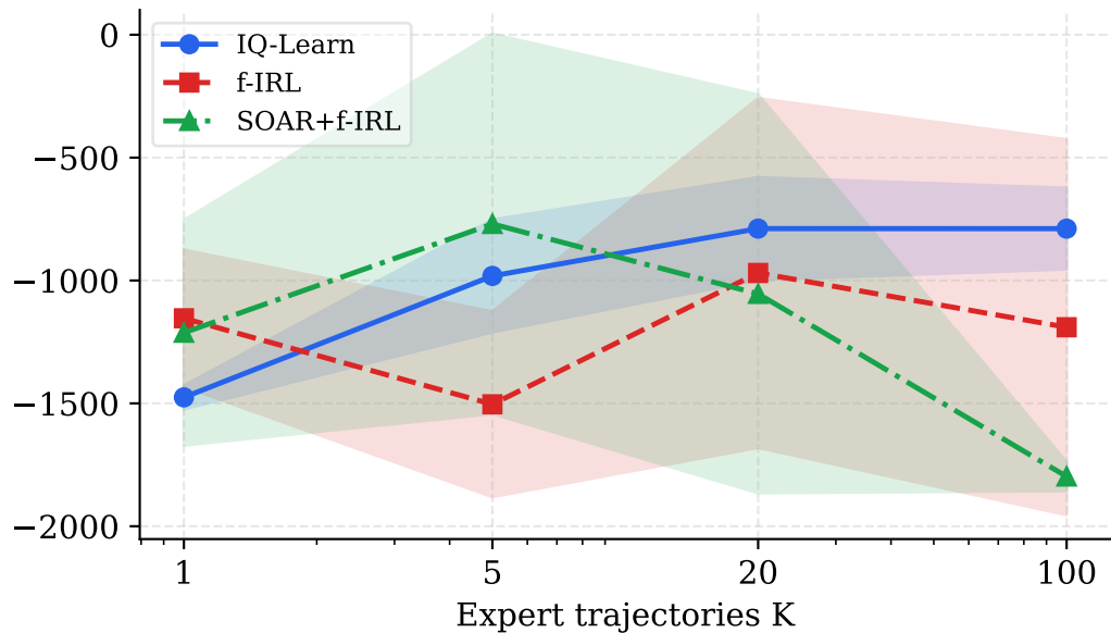
Pendulum-v1
