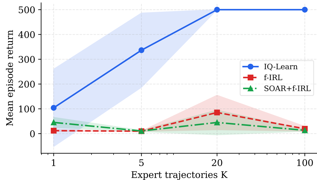
CartPole-v1
