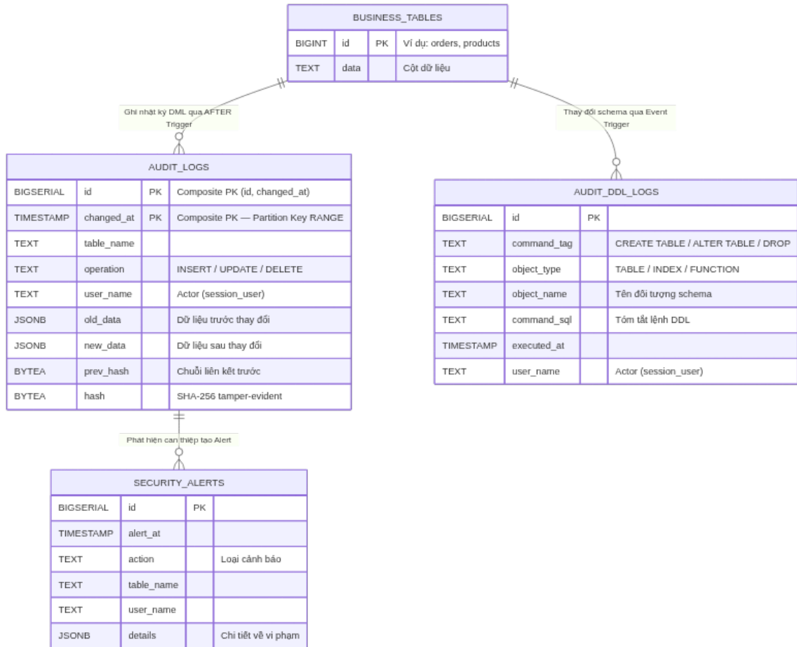
Hình 3.2. Sơ đồ thực thể (ER) hệ thống Audit Log
