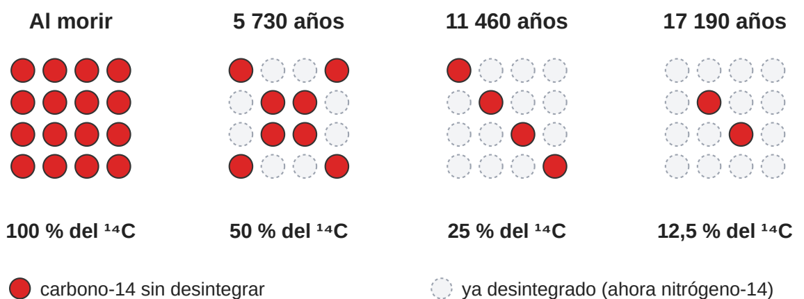
Figura 6. Los núcleos de carbono-14 de un hueso o de un trozo de madera tras la muerte. Cada 5 730 años se desintegra la mitad de los que quedaban (esquema, no a escala).
