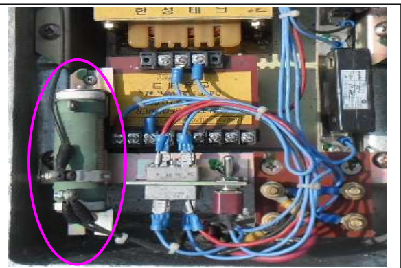
가변저항기
