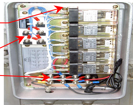
[속도조사식(s-2)제어함 내부]
