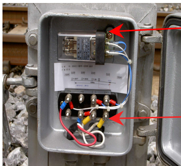
[점제어식(s-1)제어함 내부]
