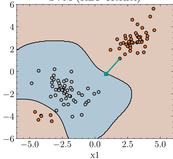
SVM (RBF Kernel)
