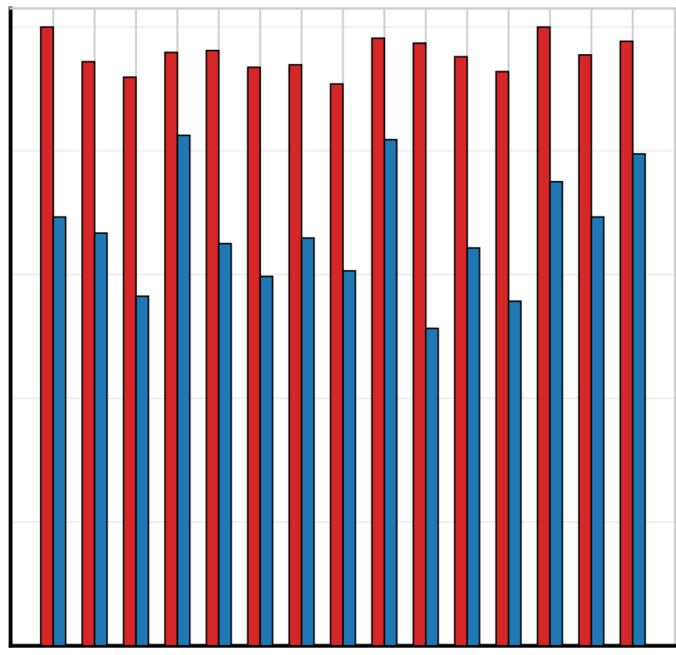
GPT-5.5
