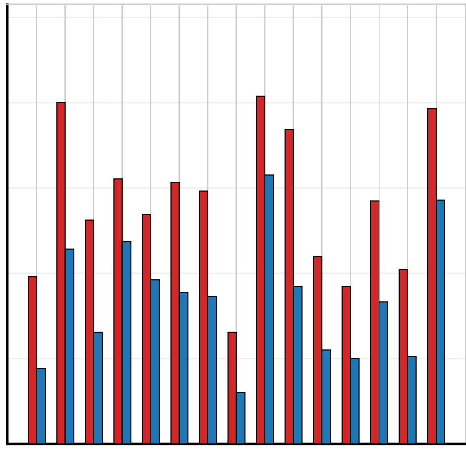
Kimi K2.5
