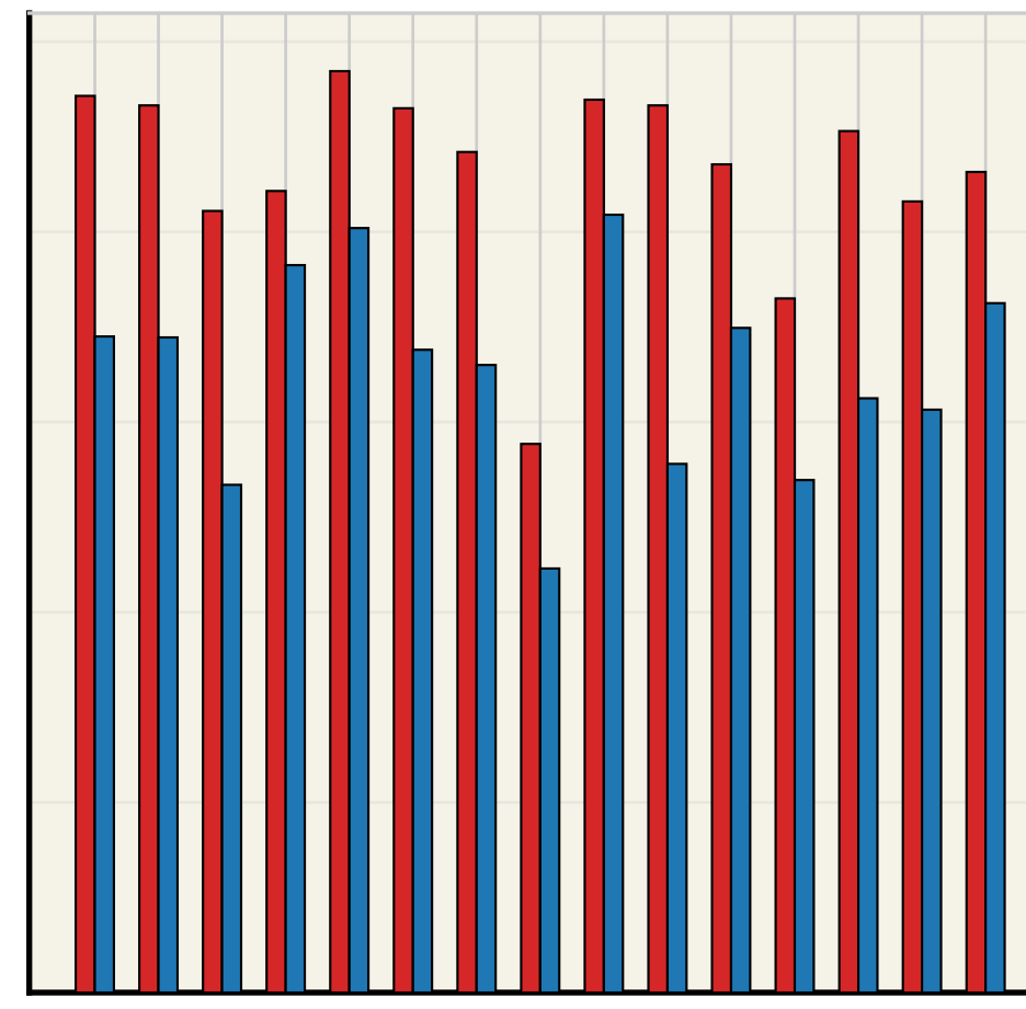
GLM-5
