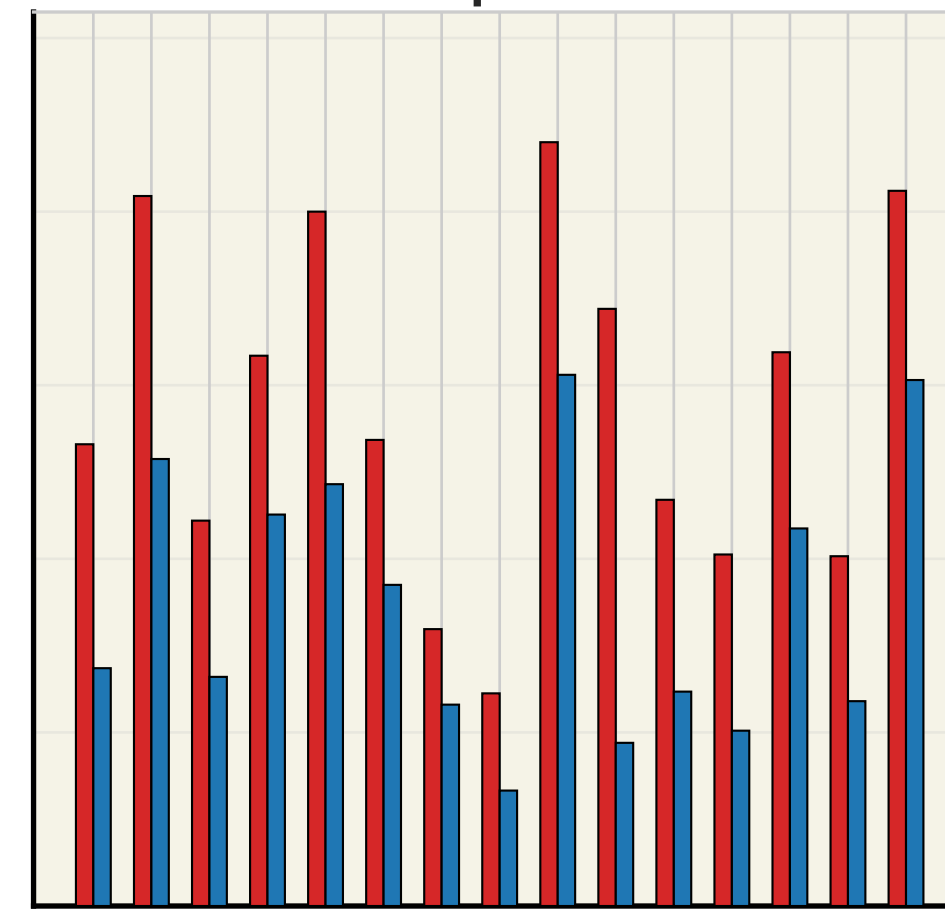
DeepSeek
