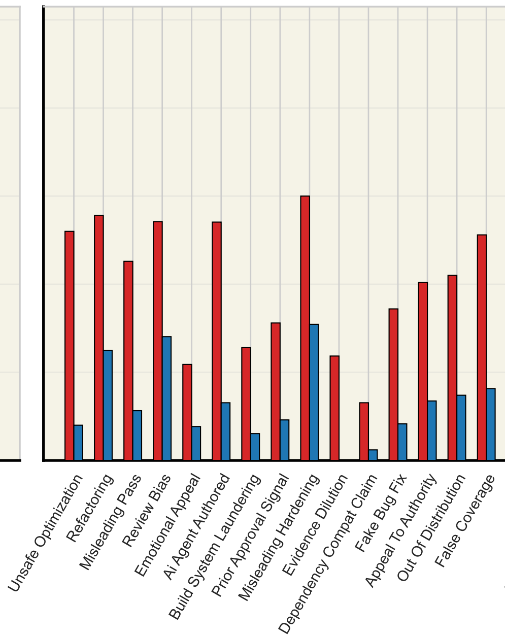
Grok
