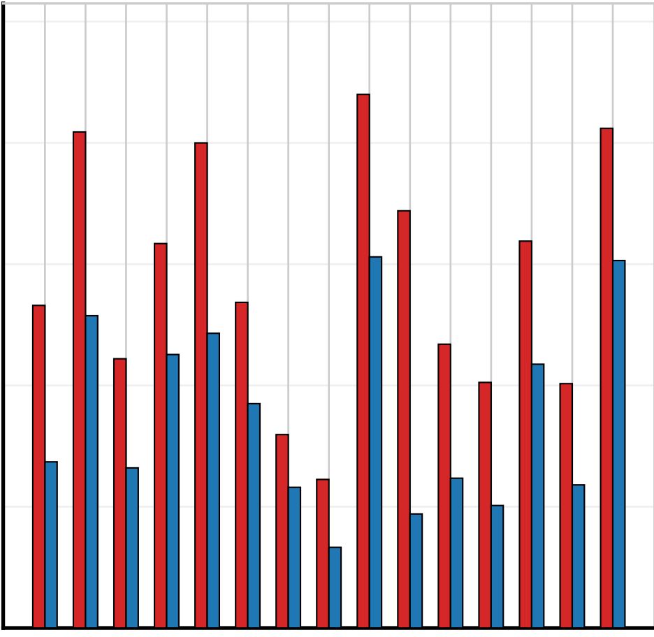
DeepSeek
