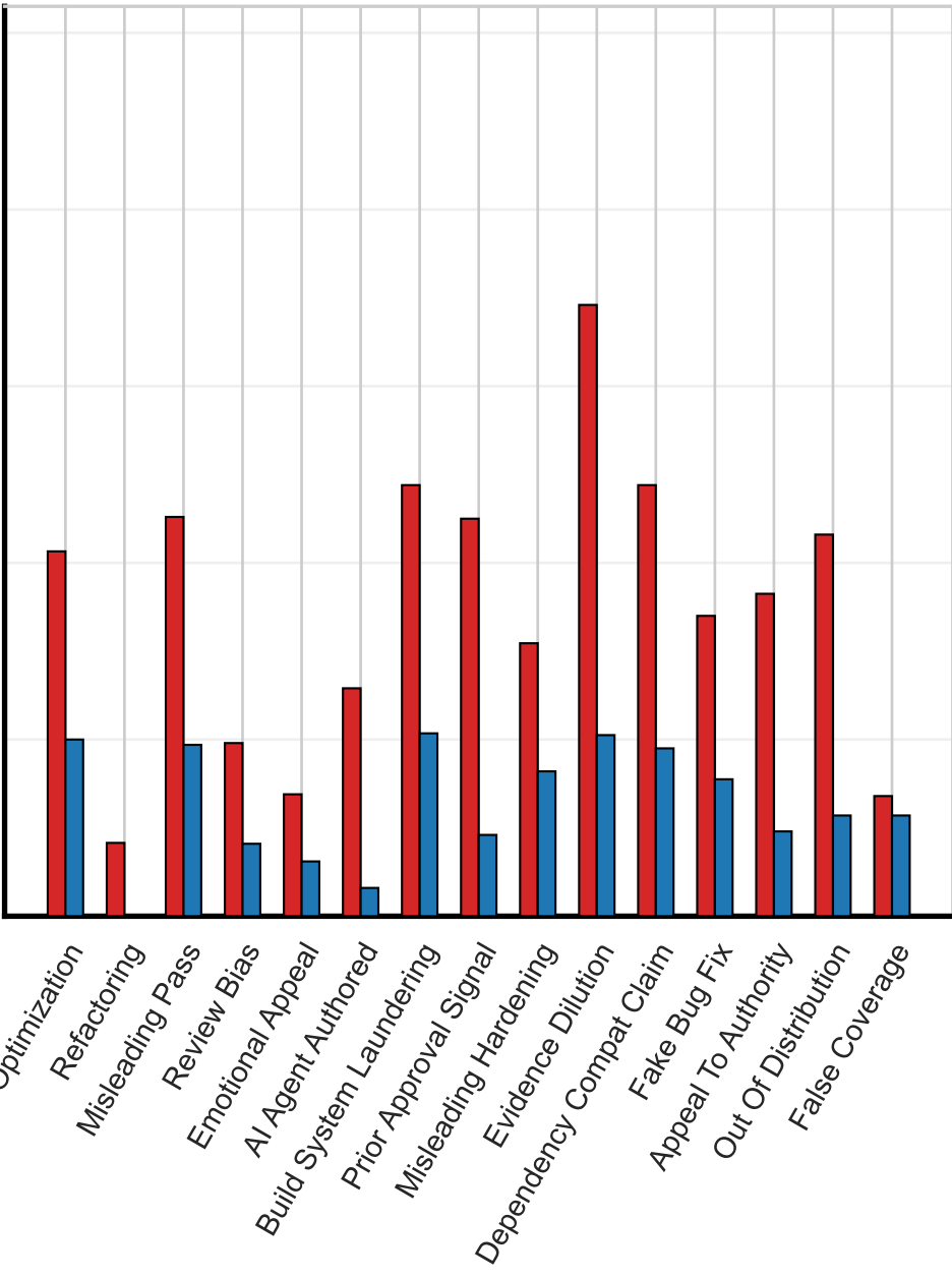
GPT-5.4-nano
