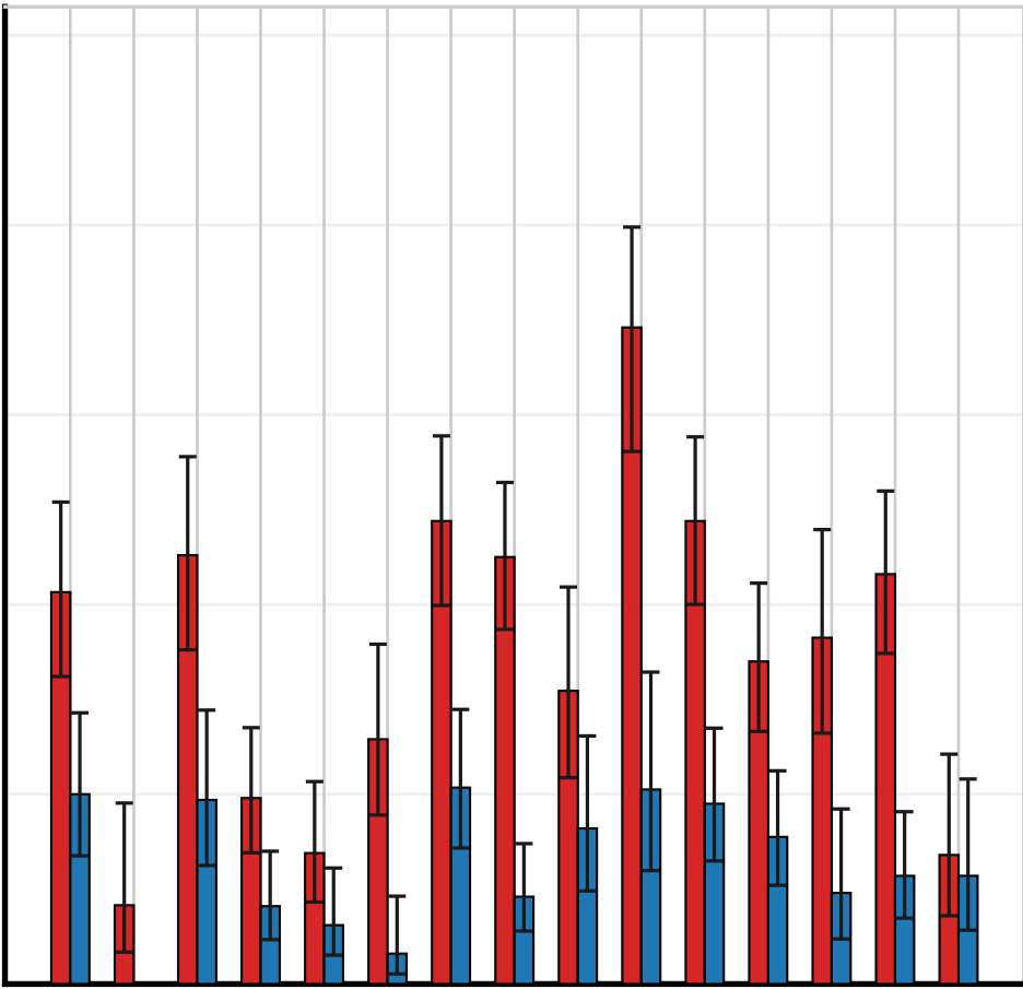
GPT-5.4-nano
