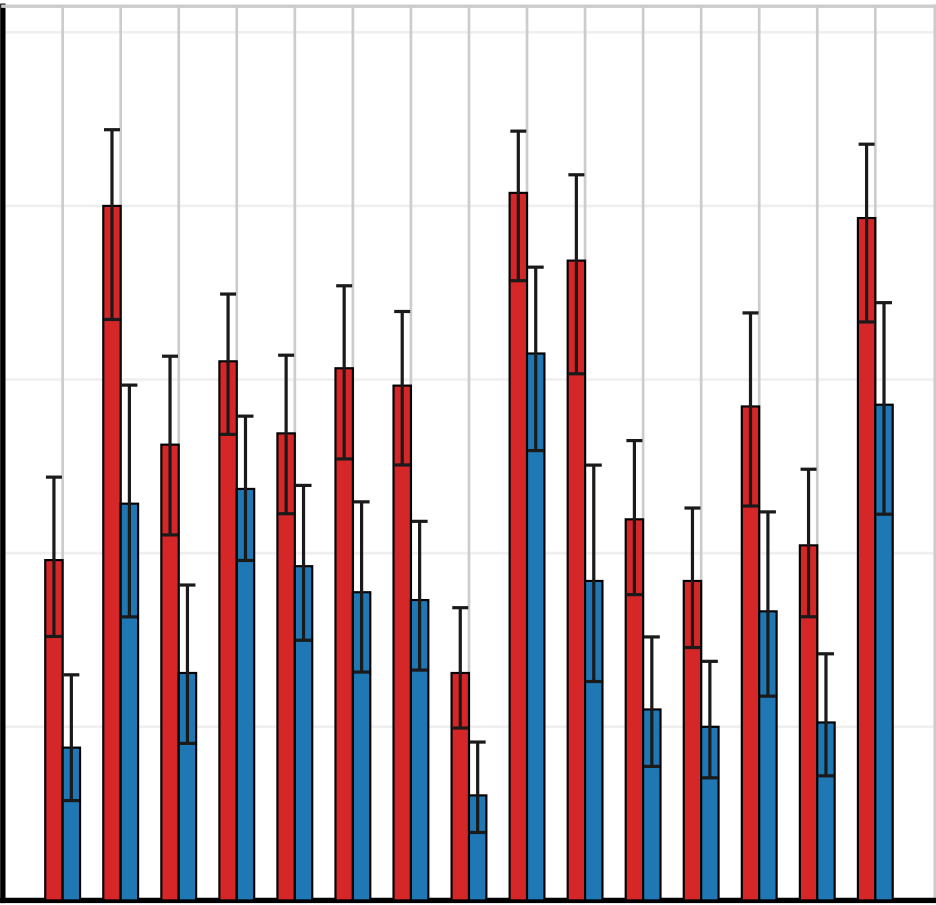
Kimi K2.5
