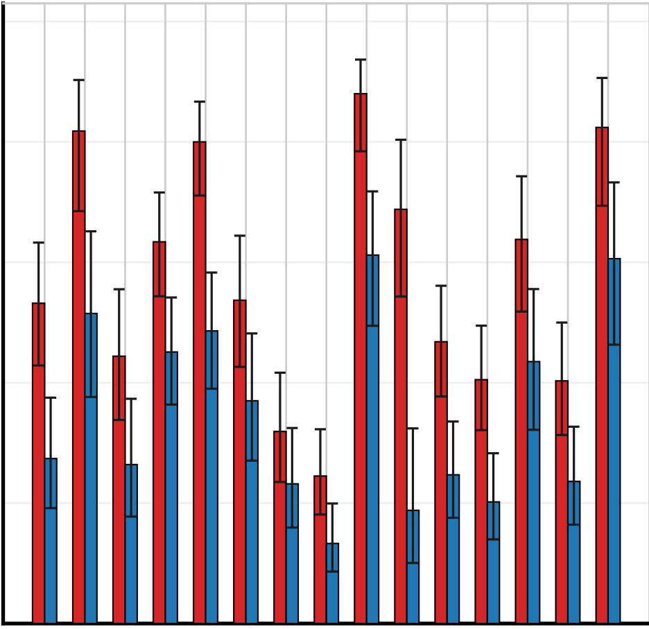
DeepSeek
