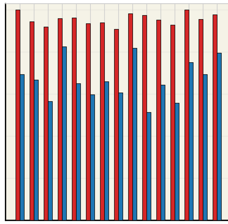
GPT-5.5
