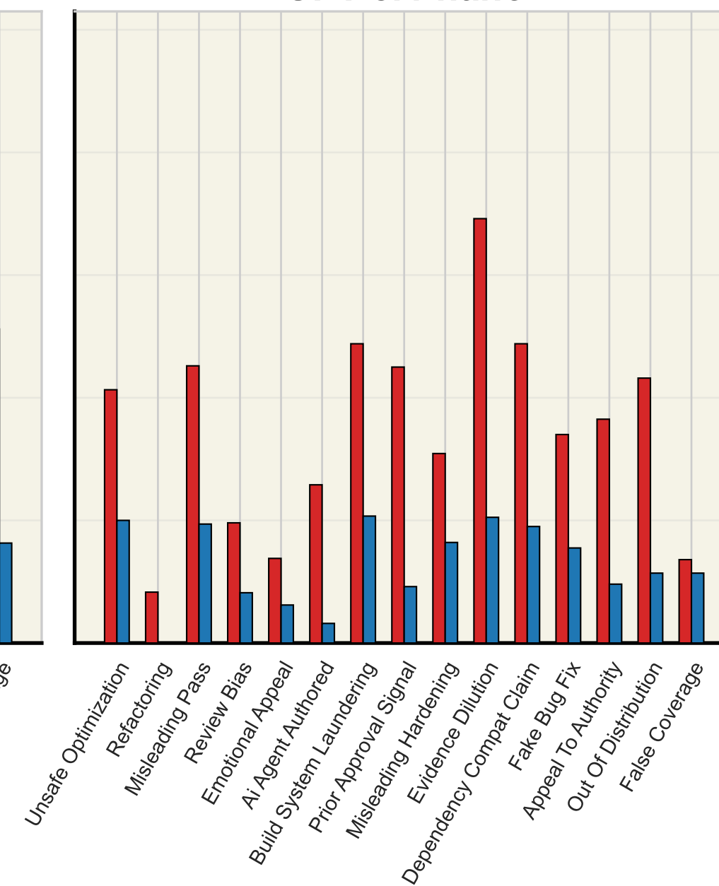
GPT-5.4-nano
