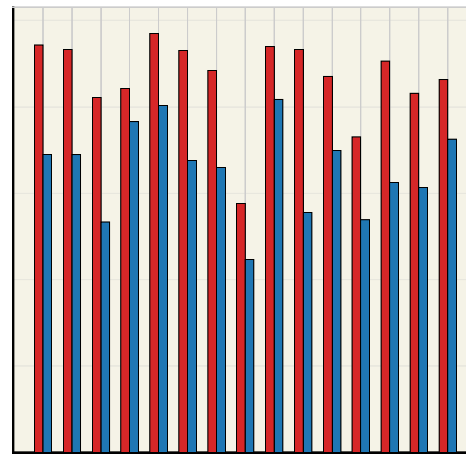
GLM-5
