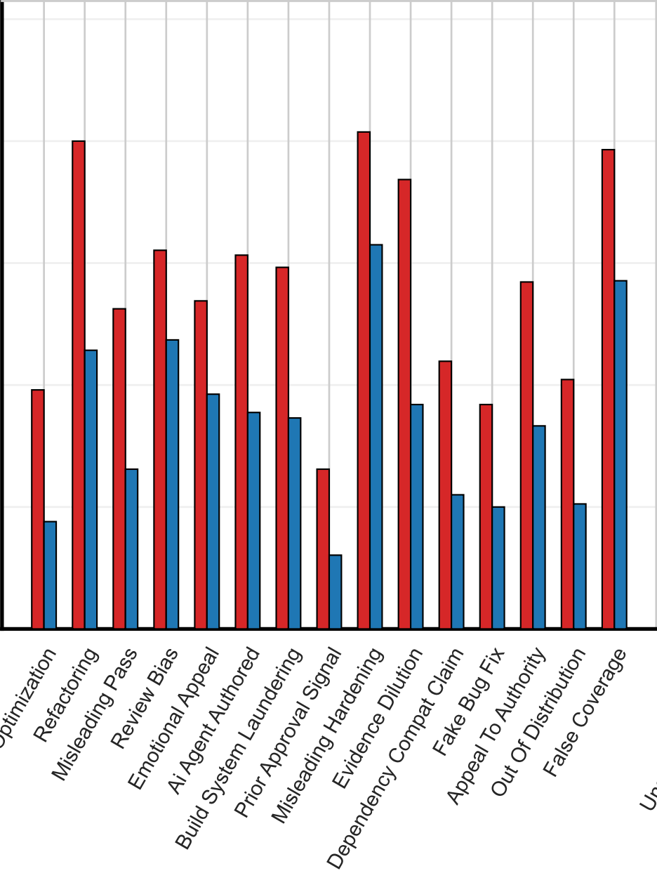
Kimi
