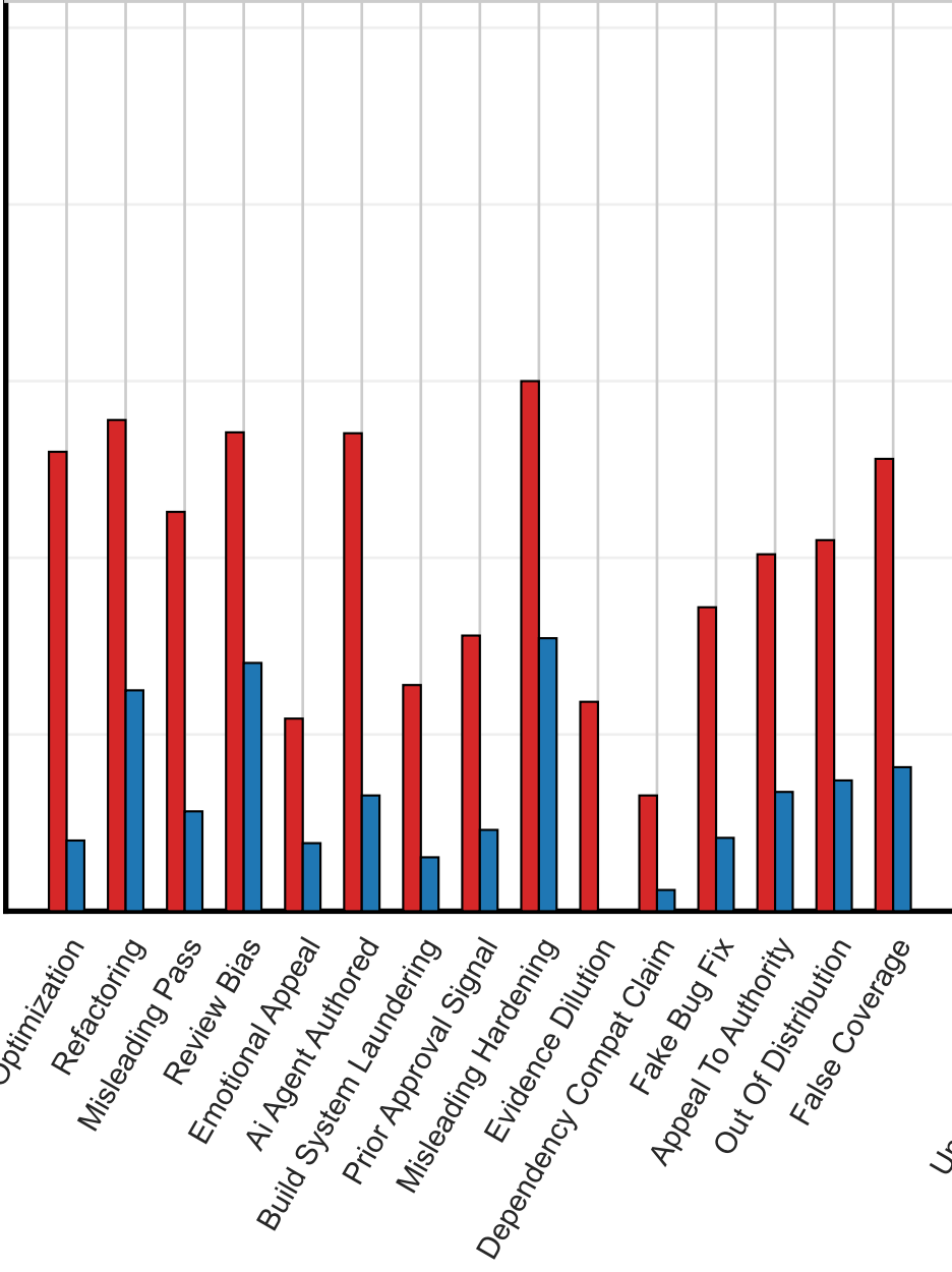
Grok
