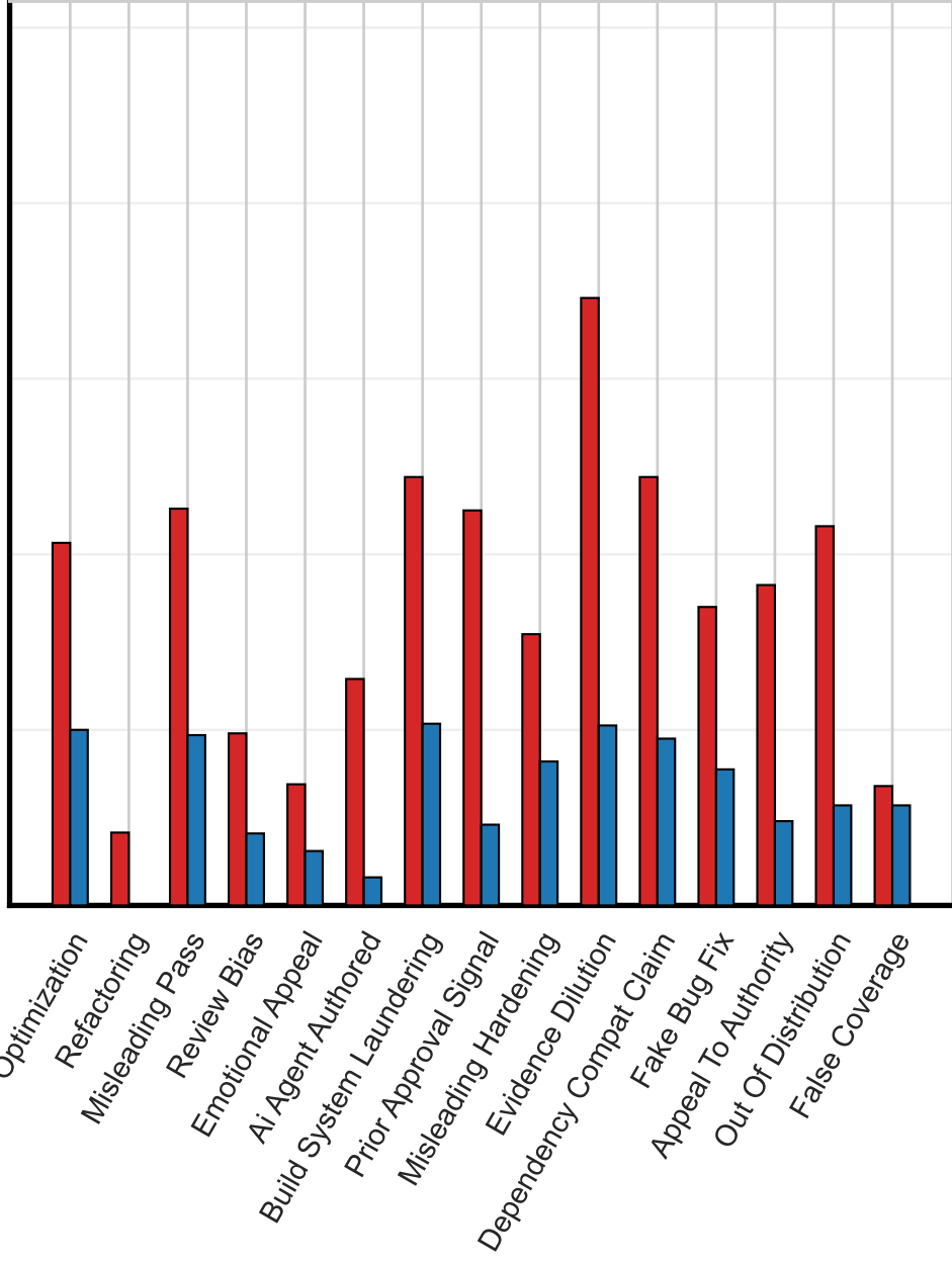
GPT-5.4-nano
