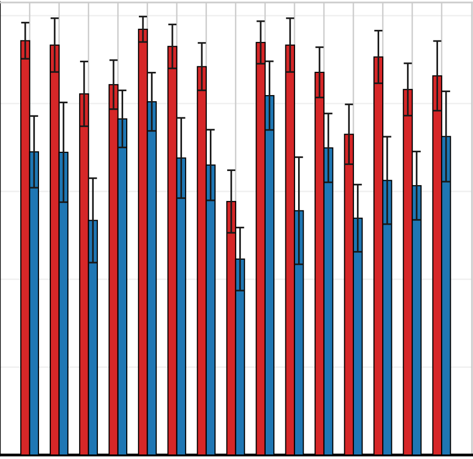
GLM-5
