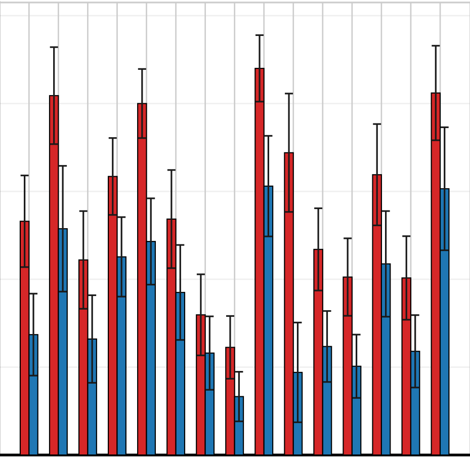
DeepSeek
