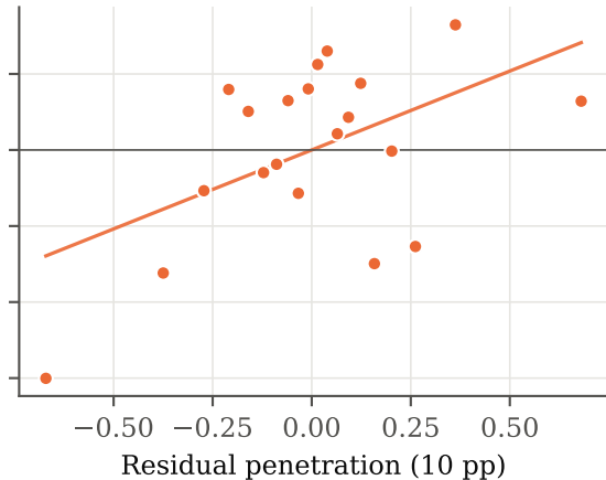
Solar: slope 4.15 per 10 pp
