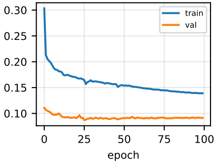
L1
