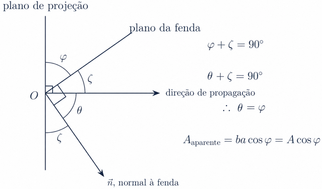
Figura 33: Relações geométricas entre o plano da fenda, o plano de projeção, a direção de propagação e a normal à fenda, usadas na determinação da área aparente.
