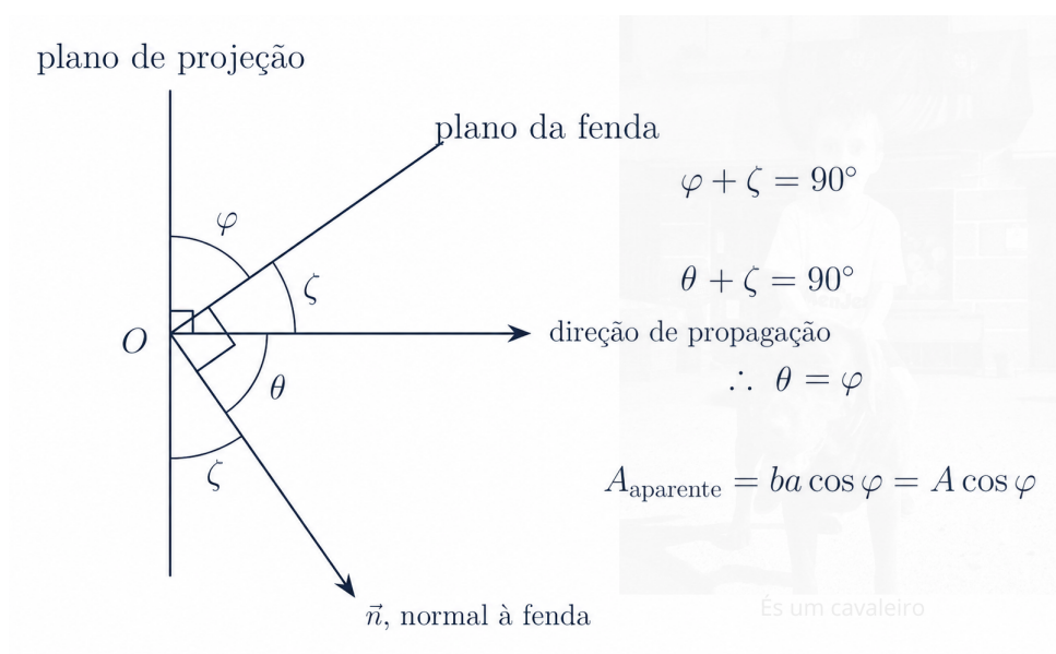
Figura 32: Projeção da fenda retangular no plano perpendicular à direção de propagação e respetiva vista frontal.
