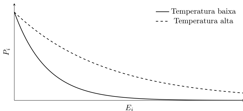
Figura 5: Comparação qualitativa entre a distribuição para uma temperatura baixa e para uma temperatura alta.
