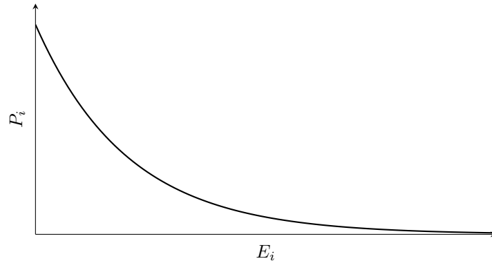
Figura 4: Comportamento qualitativo da probabilidade associada a um microestado em função da sua energia.
