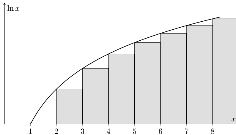
Figura 22: Interpretação do somatório como uma soma de retângulos de base 1.
