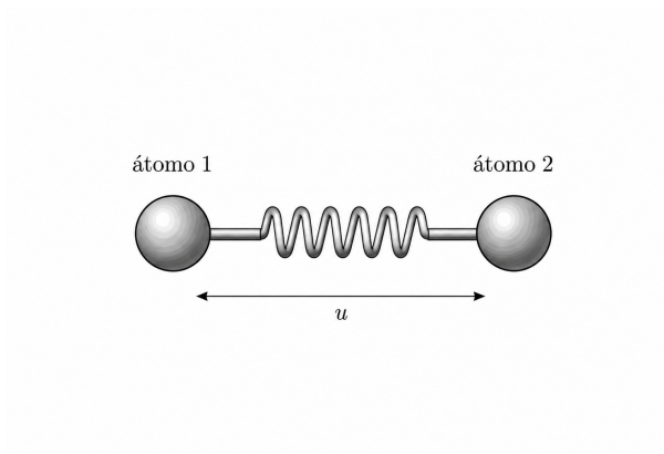
Figura 11: Representação esquemática do modo vibracional de uma molécula diatômica.
