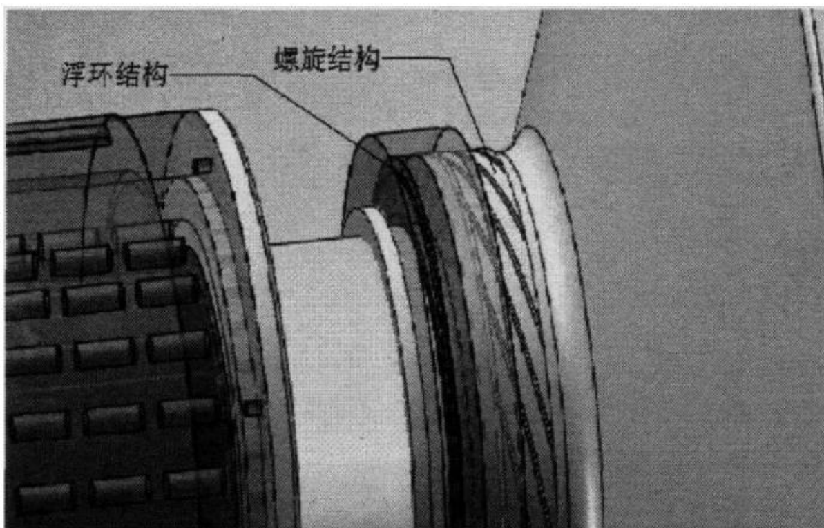
图5-3 组合式密封
