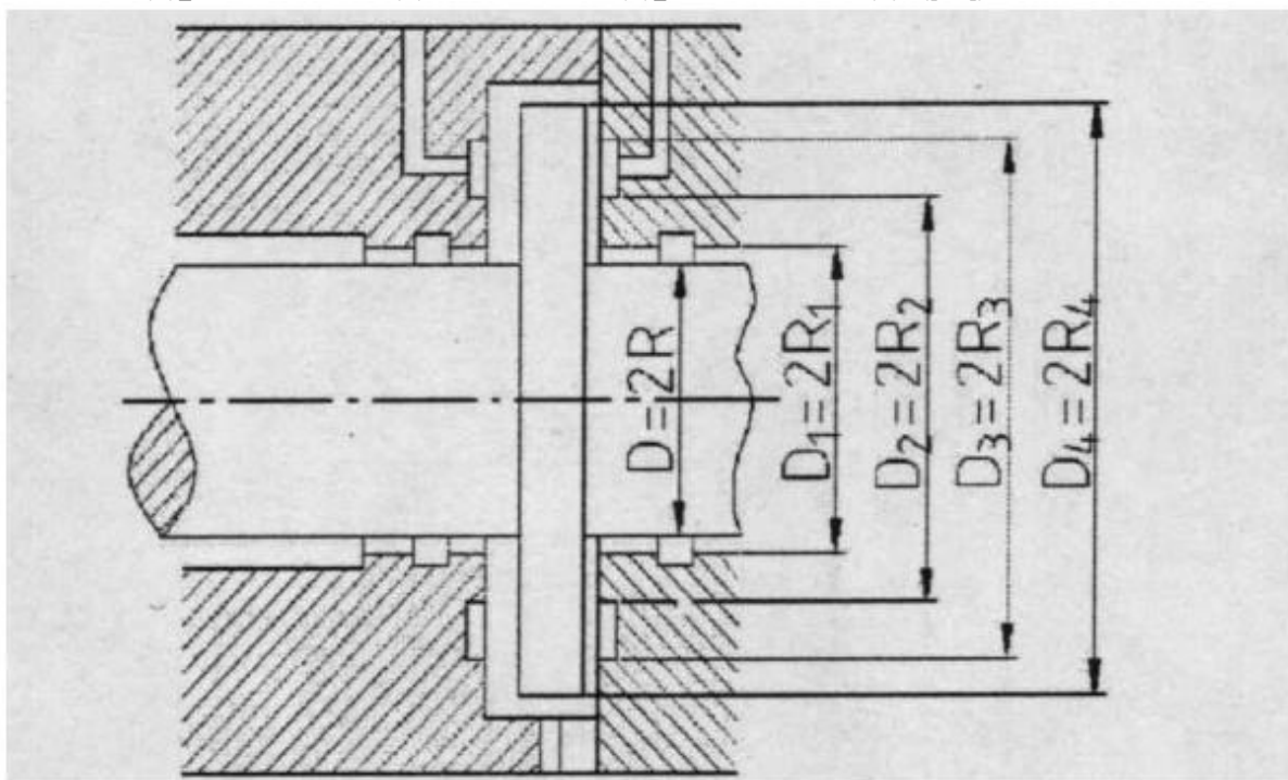
图3-10 静压轴承参数
