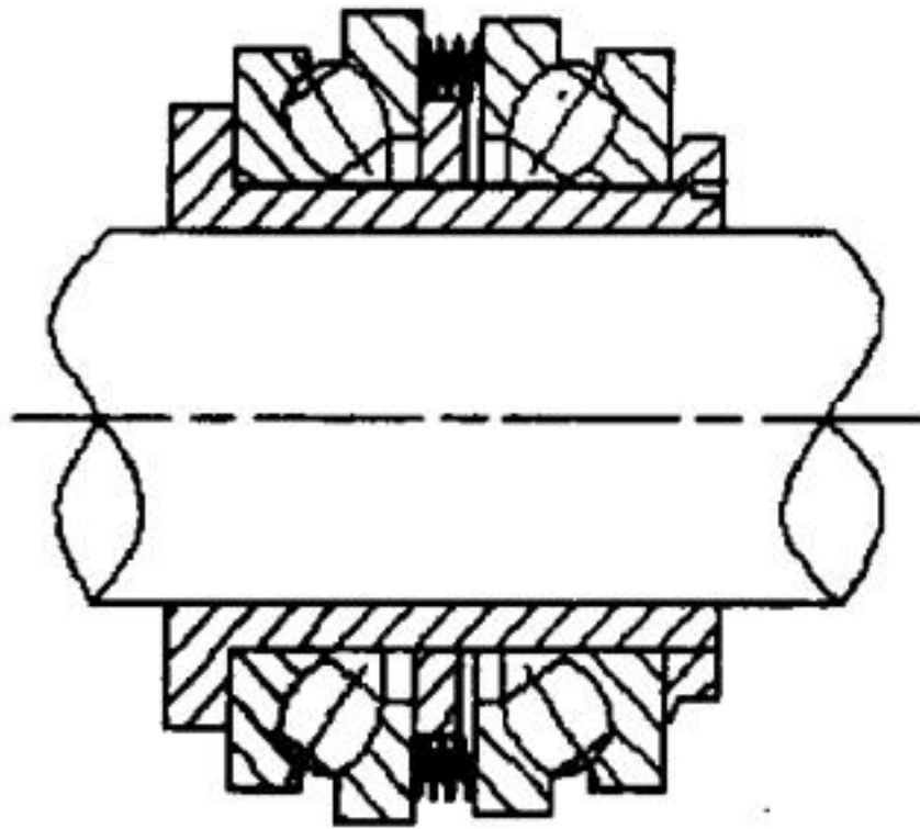
图4-1推力向心轴承
