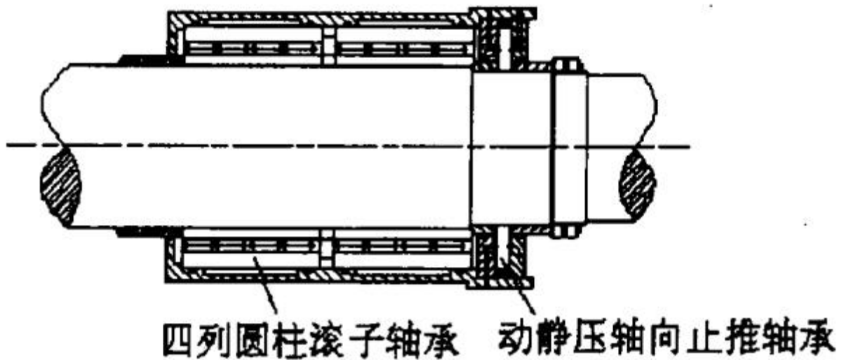
图4-1推力向心轴承
