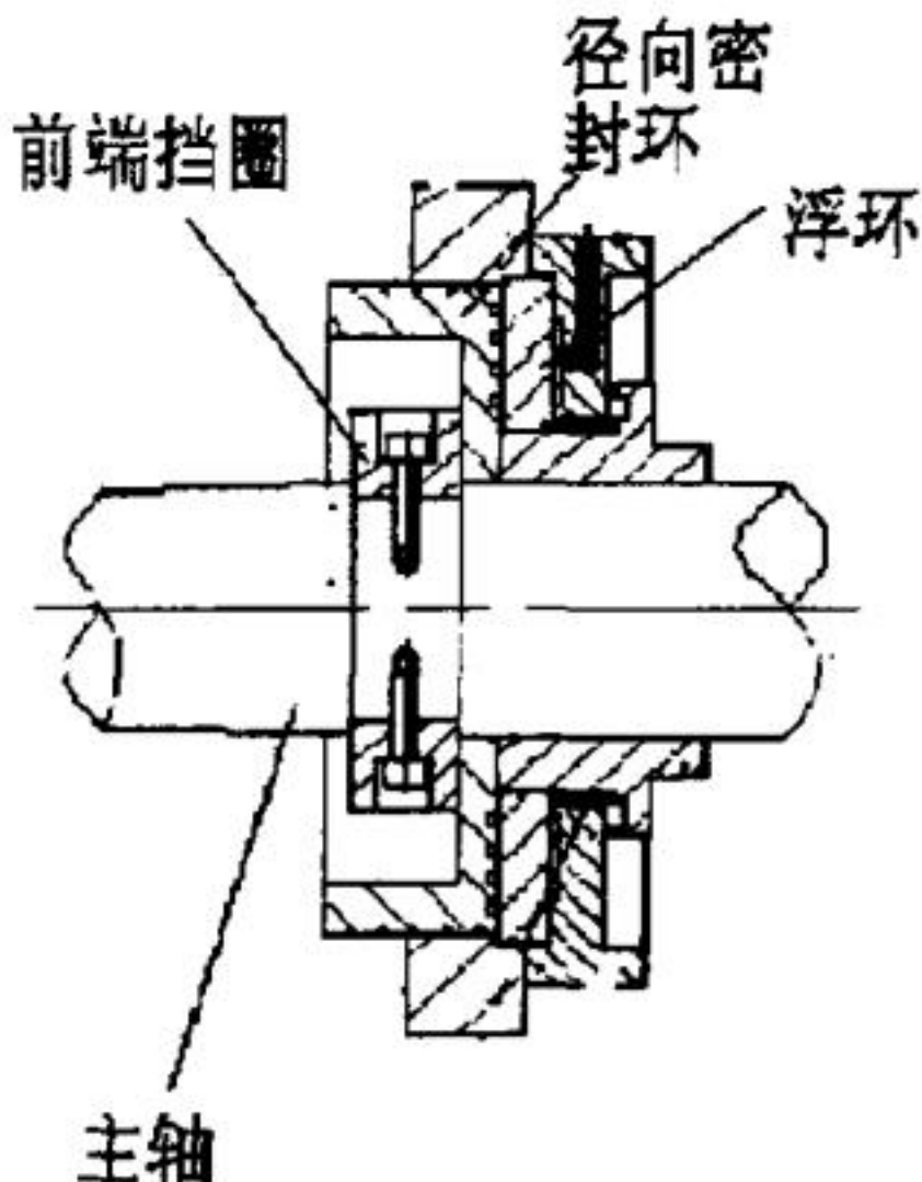
图3-16实用机械密封
