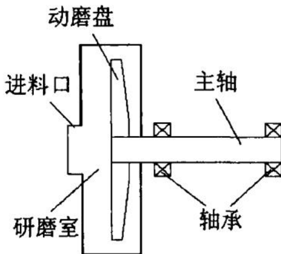
图3-1 热磨机主轴轴承支承形式
