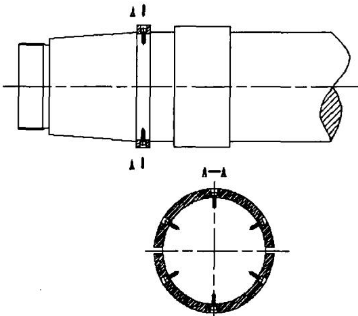
图3-3 前端主轴
