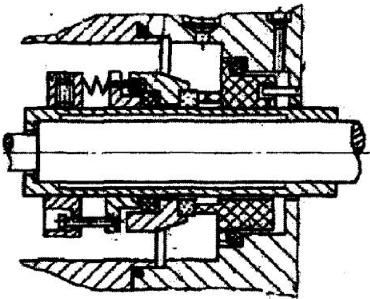
图3-15 机械密封原理图
