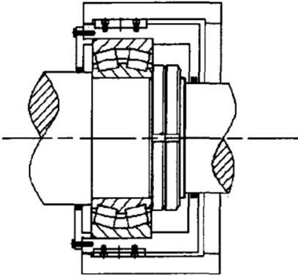
图3-9后端轴承
