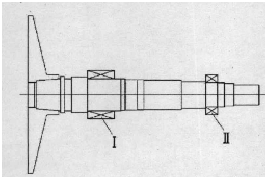
图 3-5 主轴支撑轴承
