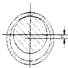
图 5-5 静止浮环最大偏心位置
