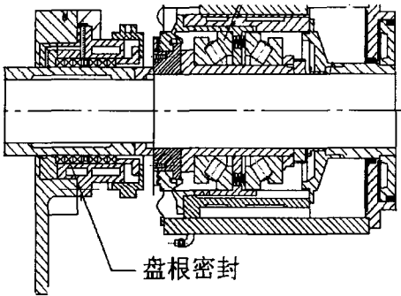
图 3-14 填料密封形式
