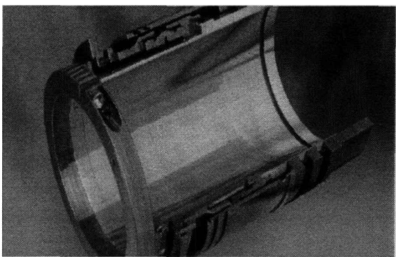
图 3-16 实用机械密封
