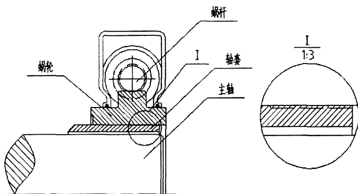
图 3-12 蜗轮蜗杆式微调结构
