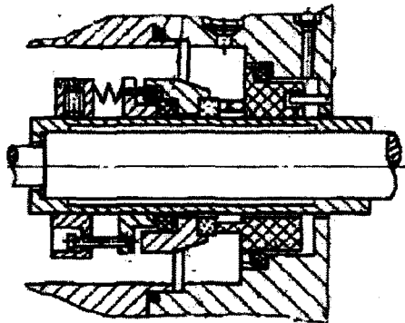
图 3-15 机械密封原理图
