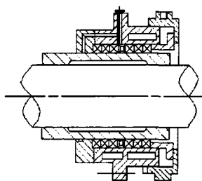
图 5-1 盘根密封结构
