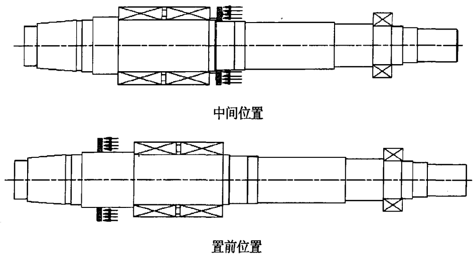
图 4-12 静压轴承的不同安装位置
