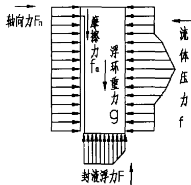
图 5-7 浮环受力示意图
