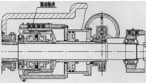
图 3-6 推力向心轴承
