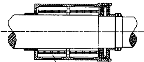
四列圆柱滚子轴承 动静压轴向止推轴承
