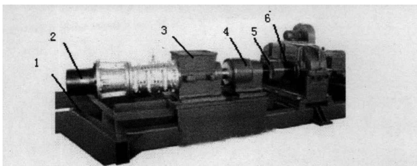
1. 底座 2. 进料电机 3. 轴承箱 4. 进料螺旋 5. 外塞管 6. 内塞管
