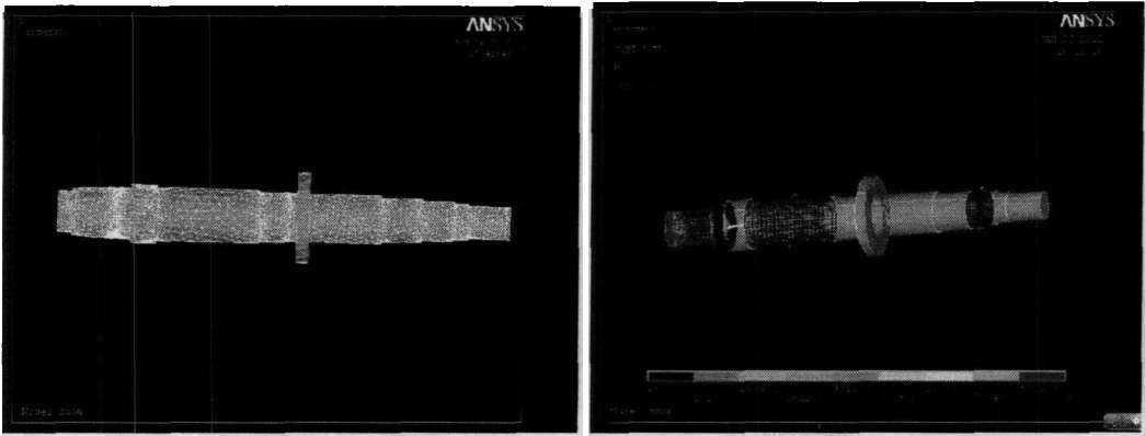
图 4-9 网格单元图
