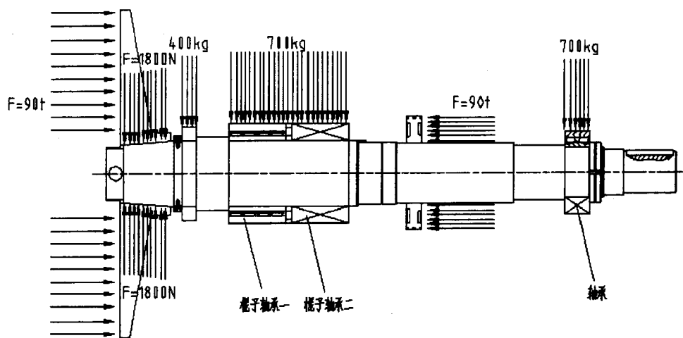
图 4-7 热磨机主轴受力分析
