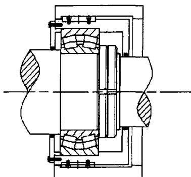
图 3-9 后端轴承
