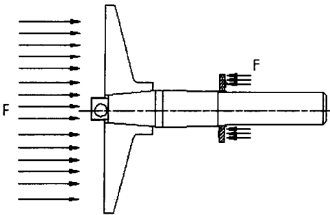
图 4-3 热磨机静压轴承位置
