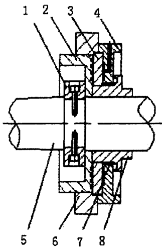
1. 卡环 2. 动环 3. 浮环 4. 进液环 5. 轴 6. 壳体 7. 密封圈 8. 轴套
