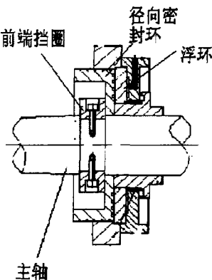
图 3-17 机械式径向浮环密封
