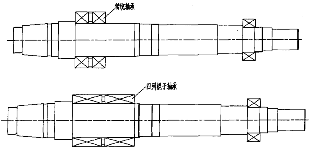
图 4-6 热磨机两种轴承形式
