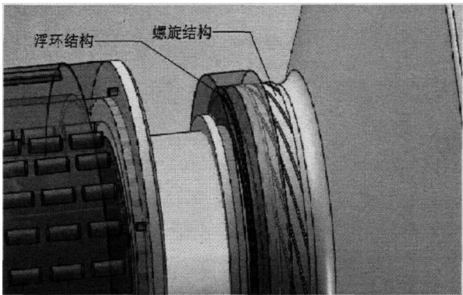
图 5-3 组合式密封
