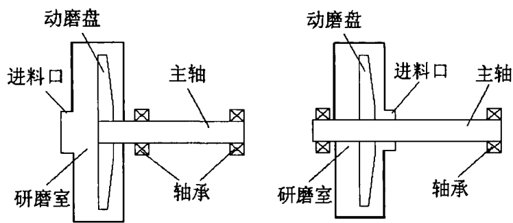
图 3-1 热磨机主轴轴承支承形式
