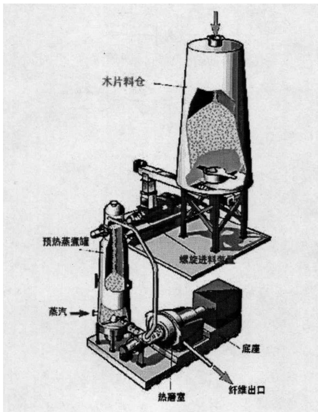
图 2-7 热磨机主要部件
