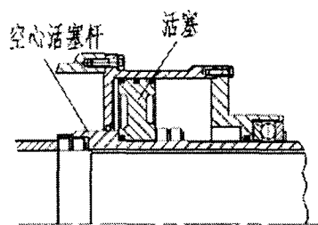
图 3-13 液压缸装置
