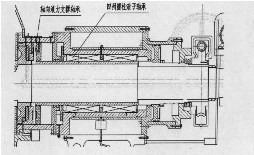
图 3-8 新组合轴承形
