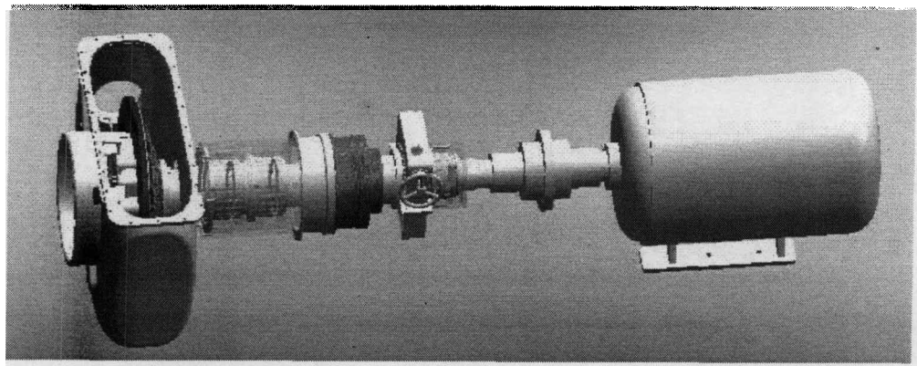
图 6-3 主机的装配图
