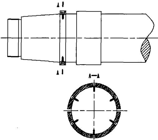
图 3-3 前端主轴
