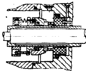
图 5-2 机械密封结构
