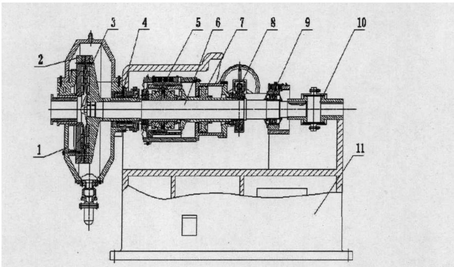
1. 研磨室体 2. 固定磨盘 3. 动磨盘 4. 密封装置 5. 前轴承组 6. 主轴 7. 液压缸 8. 微调装置 9. 后轴承组 10. 联轴器 11. 箱体
