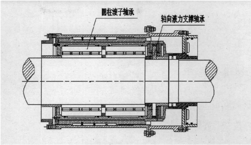
图 4-5 静压轴承中置式
