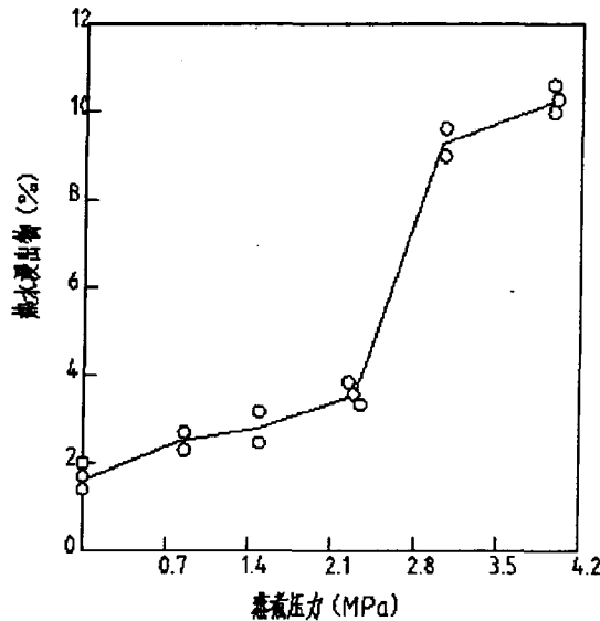
图 2-4 蒸煮预热压力与纤维热水抽出物的关系
