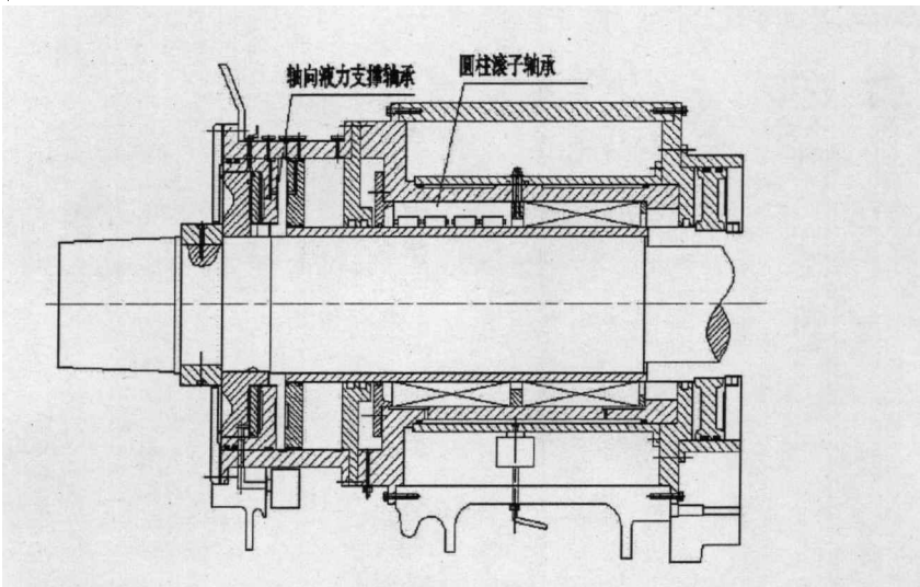
图 4-4 静压轴承前置式
