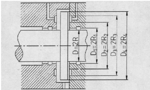
图 3-10 静压轴承参数
