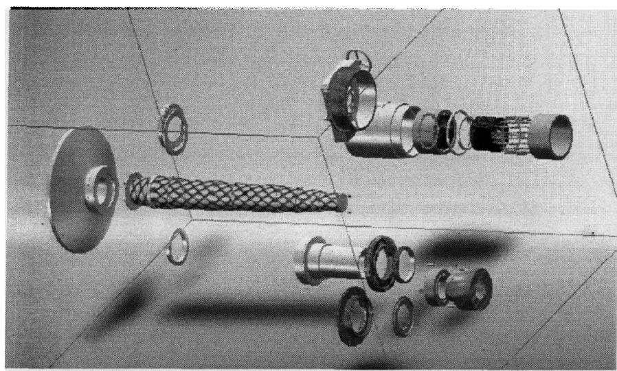
图 6-2 主轴零部件爆炸图
