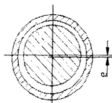
图 5-6 工作浮环最小偏心位置
