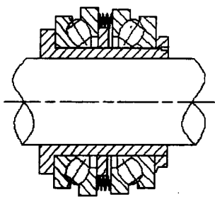
图 4-1 推力向心轴承
