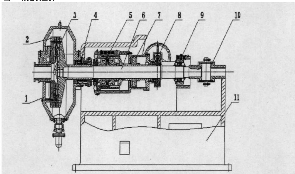
图2-9 热磨机主机
