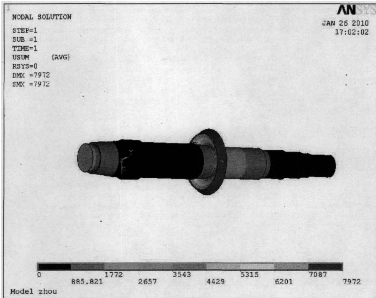
图4-10位移云图
