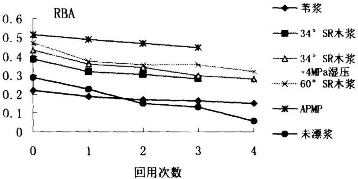
图2-15RBA随回用的变化关系
