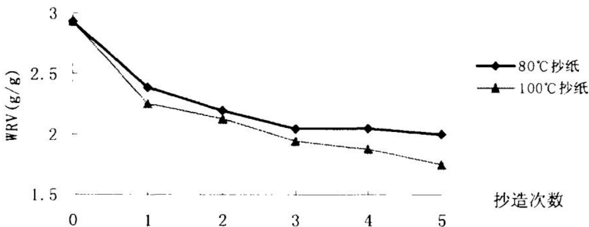
图3-4不同干燥温度苇浆保水值随回用变化
