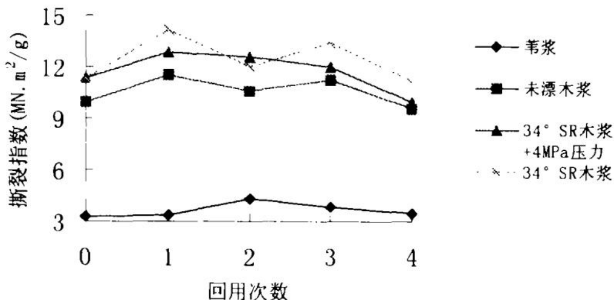
图2-10 撕裂度与回用次数的关系
