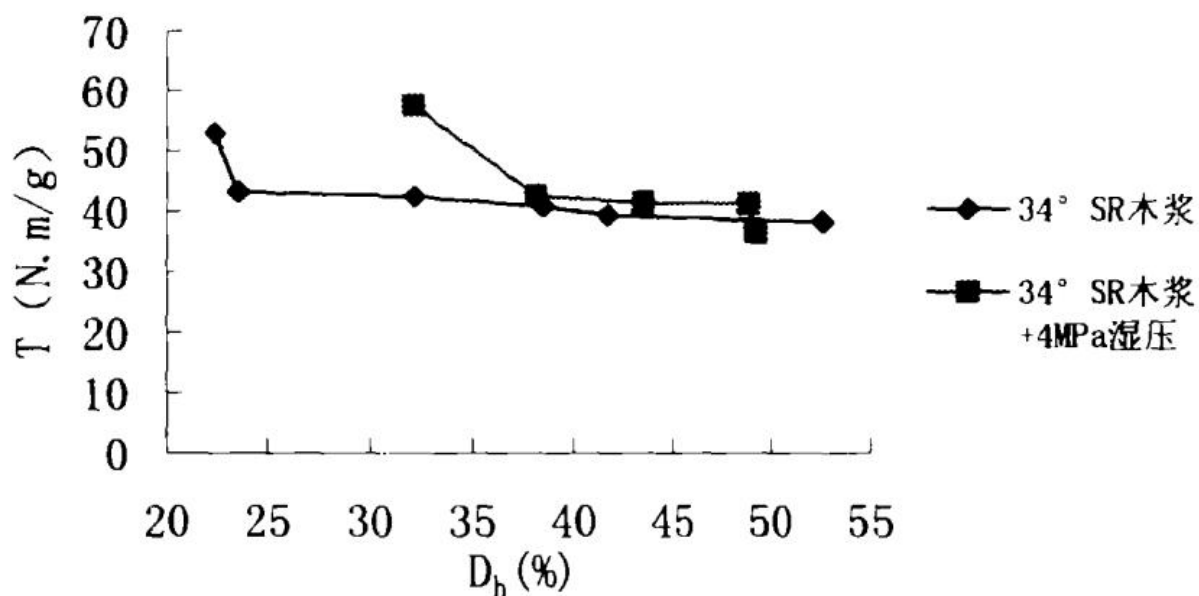
图5-1木浆纤维损伤与纸页强度的关系
