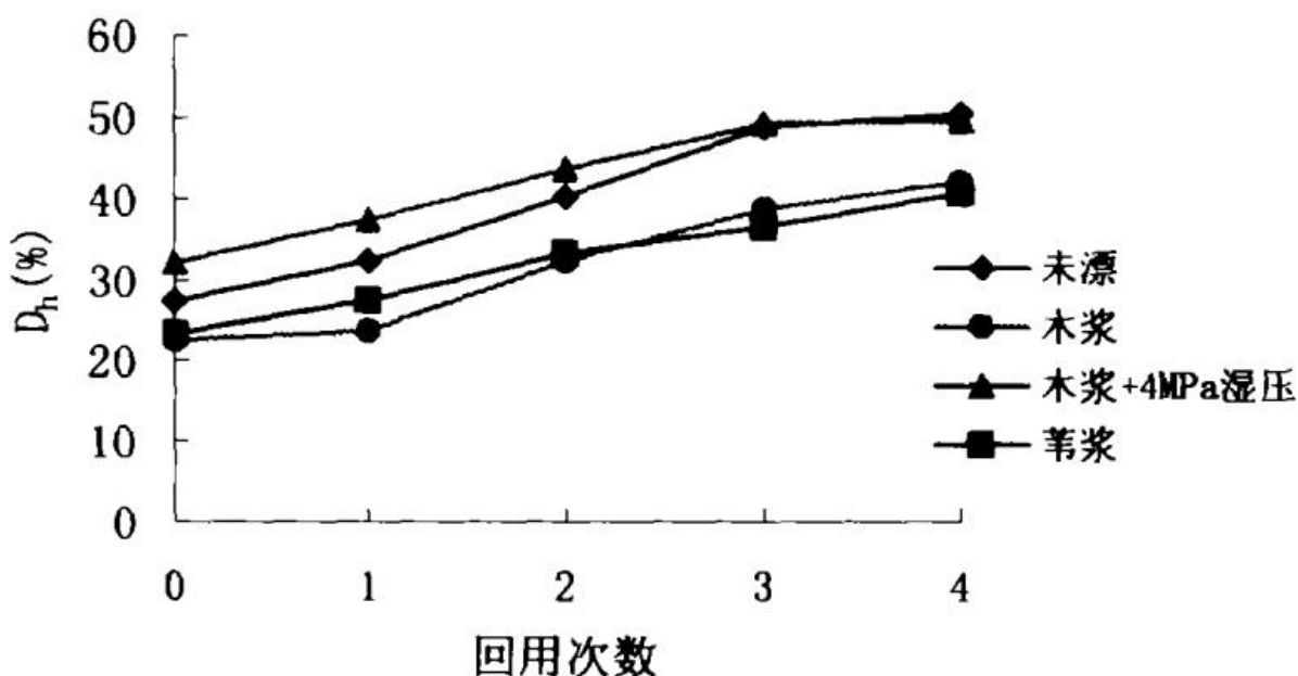
图5-4纤维损伤随回用的变化
