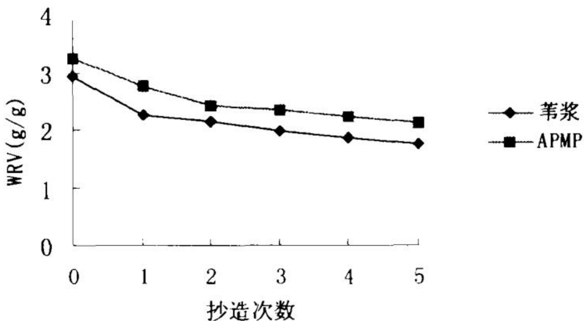
图2-4保水值与抄造次数的变化关系
