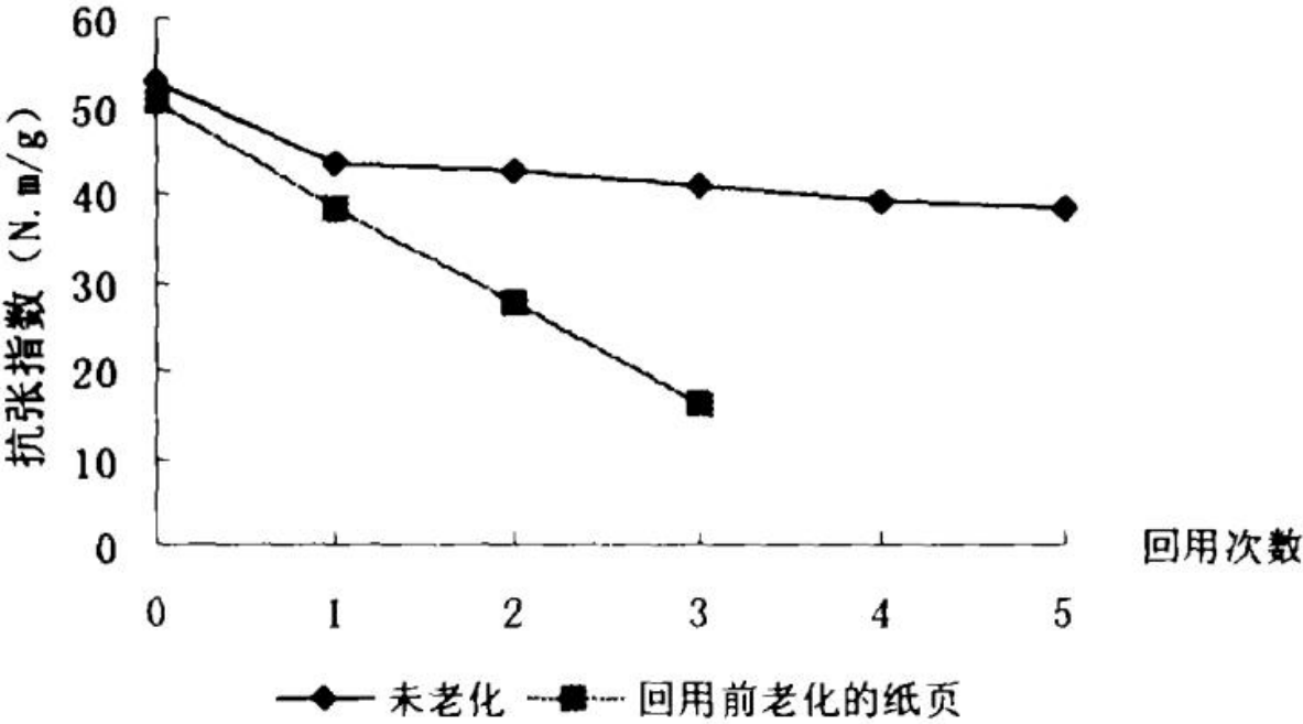
图5-9回用过程中老化损伤变化
