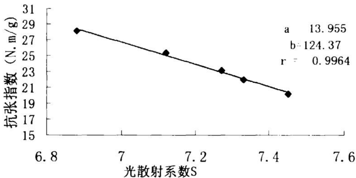
图2-12苇浆抗张强度与光散射系数曲线
