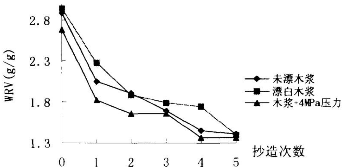
图2-5木浆WRV与回用的关系
