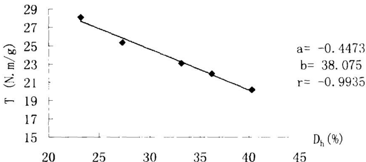
图5-3苇浆纸页强度随纤维损伤的变化
