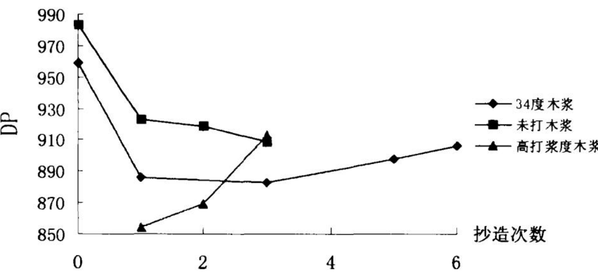
图2-1 回用过程中木浆DP的变化
