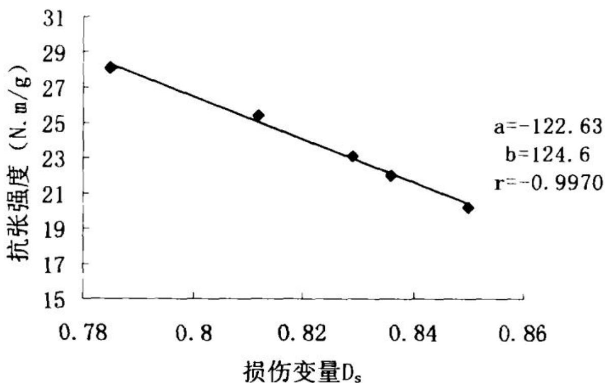
图5-5苇浆纤维损伤与成纸抗张强度的关系
