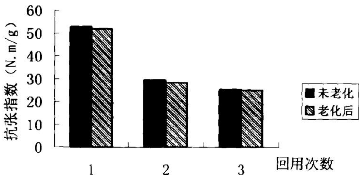
图5-11纸页老化回用损伤变化曲线
