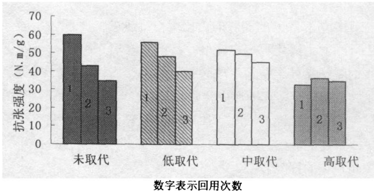
图4-4羧甲基化后纸页强度随回用的变化
