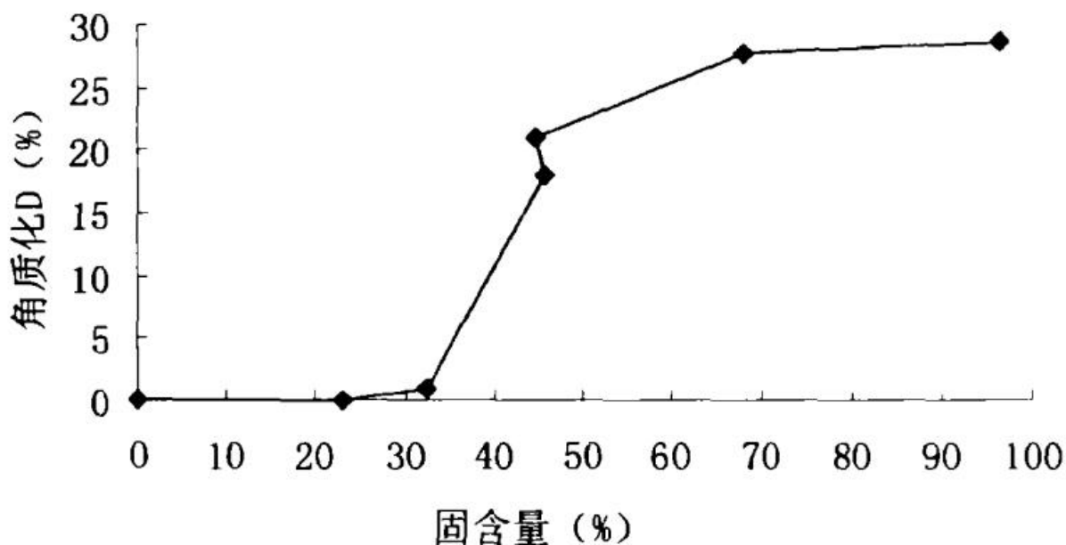
图3-2干燥过程中纤维角质化损伤的发展
