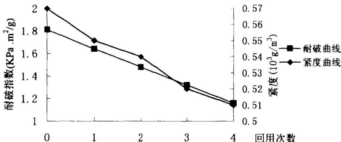
图2-9纸页紧度和耐破与回用的关系
