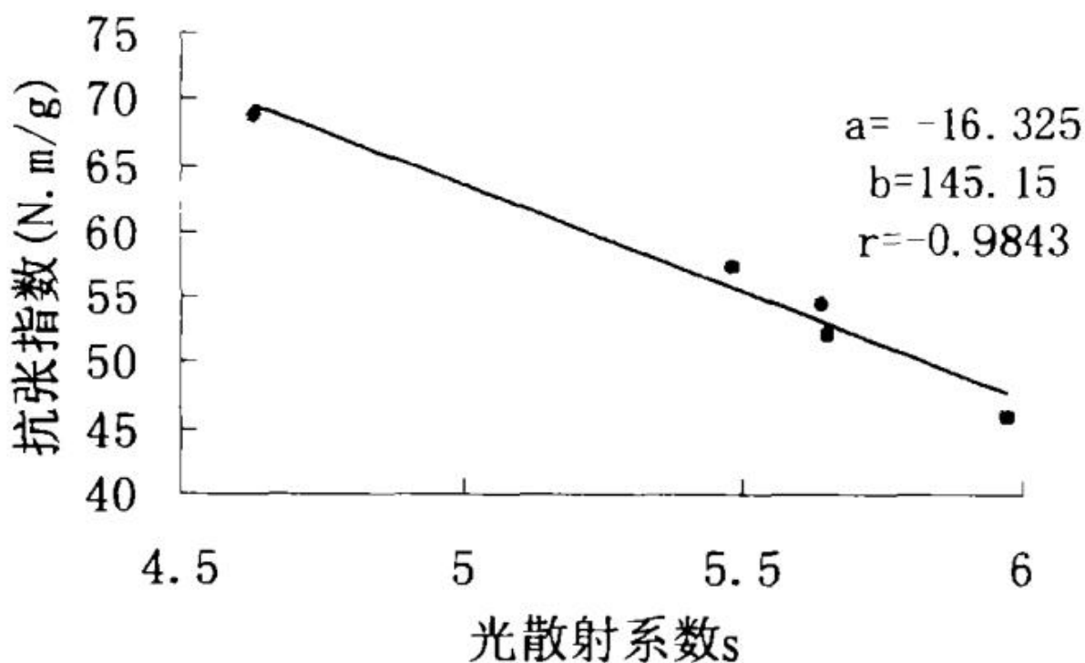
图2-13木浆抗张强度与光散射系数的关系
