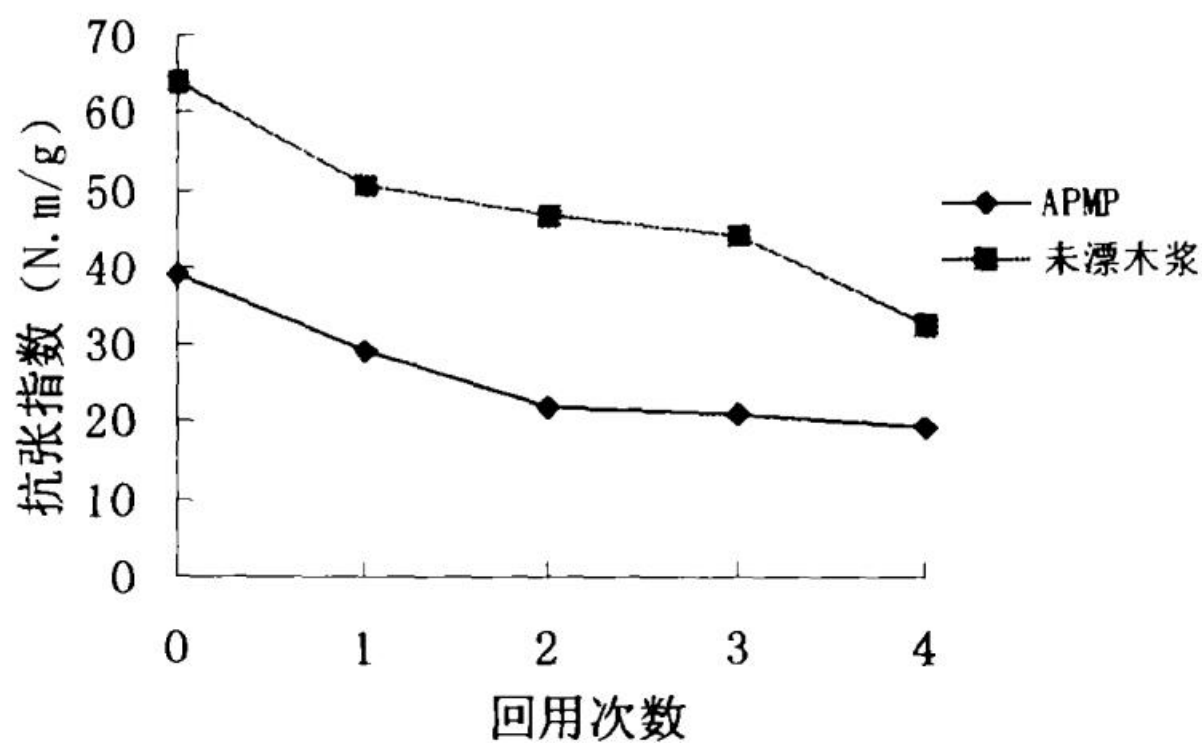
图2-8回用对纸页抗张强度的影响
