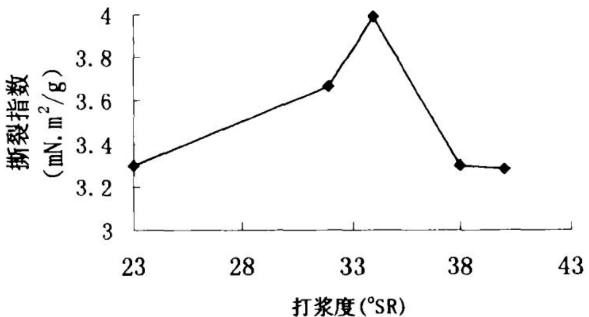
图2-11苇浆撕裂度与打浆度的关系
