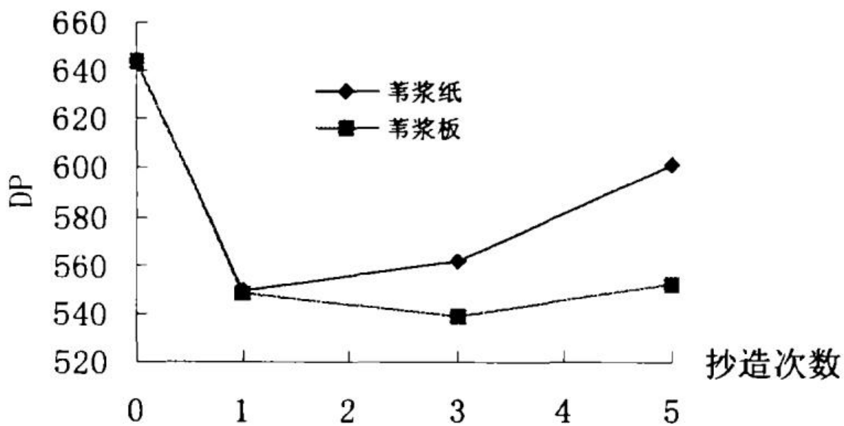
图2-2回用对苇浆DP的影响
