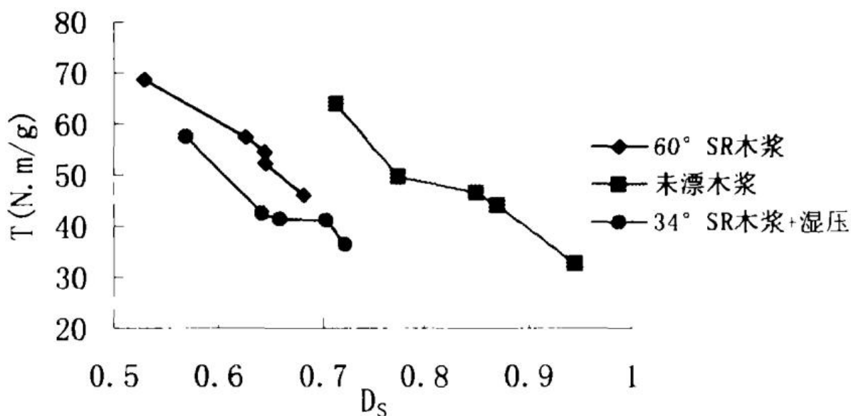
图5-6木浆纸页随纤维损伤的变化
