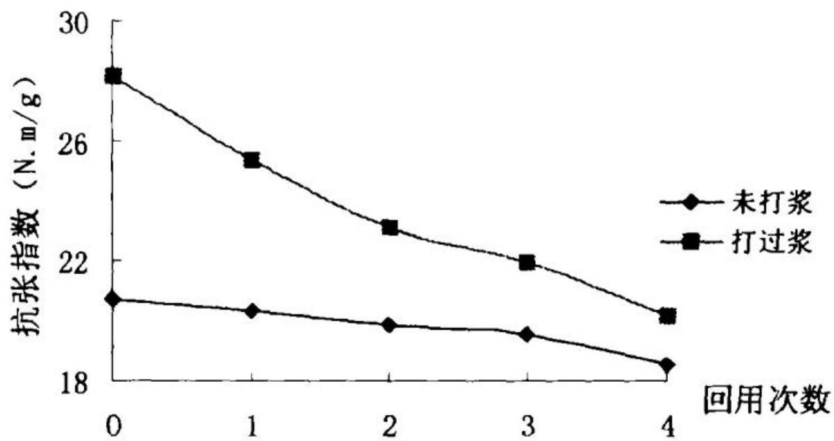
图2-7苇浆抗张强度随回用次数的变化
