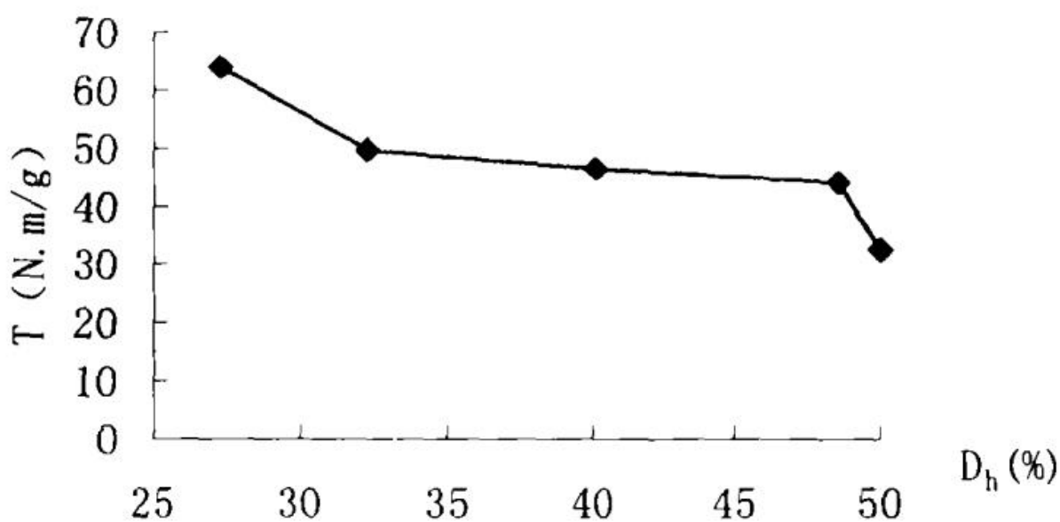
图5-2未漂木浆损伤与纸页强度关系
