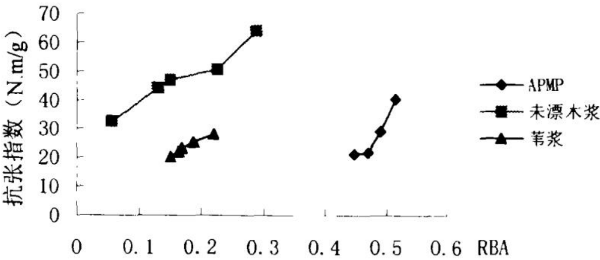
图2-14相对键合面积与抗张强度的变化关系
