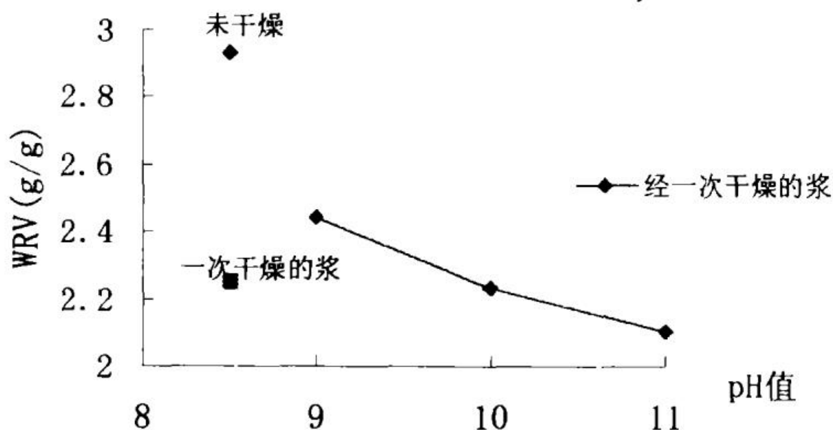
图3-5抄造环境对纤维角质化的影响
