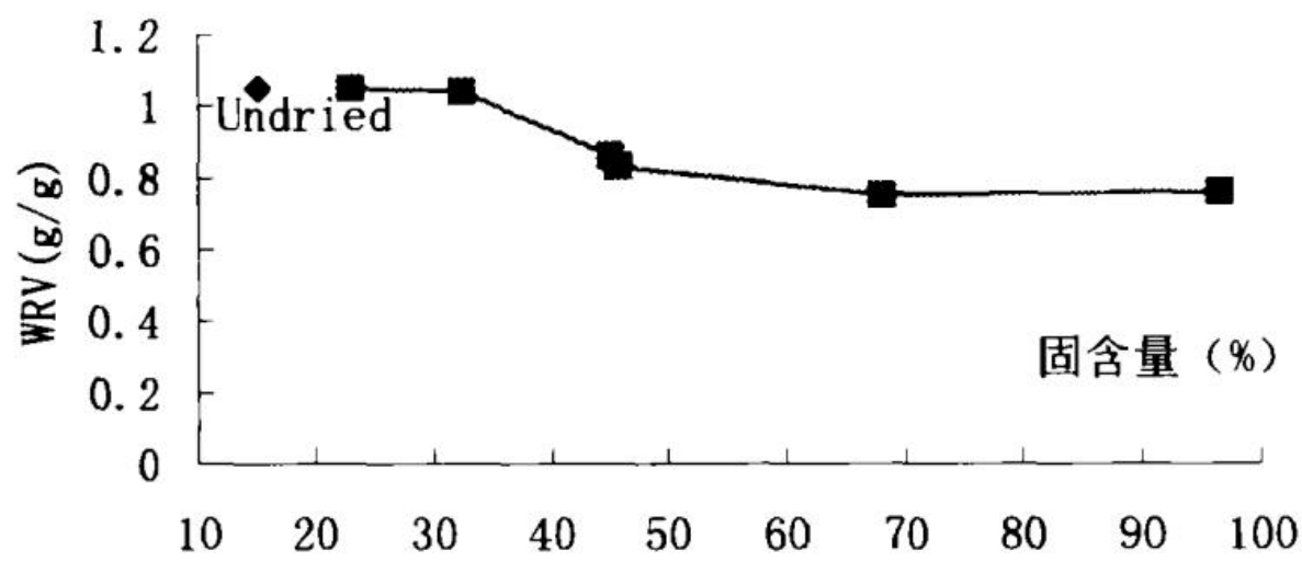
图3-1 未打木浆干燥中固含量与保水值的变化
