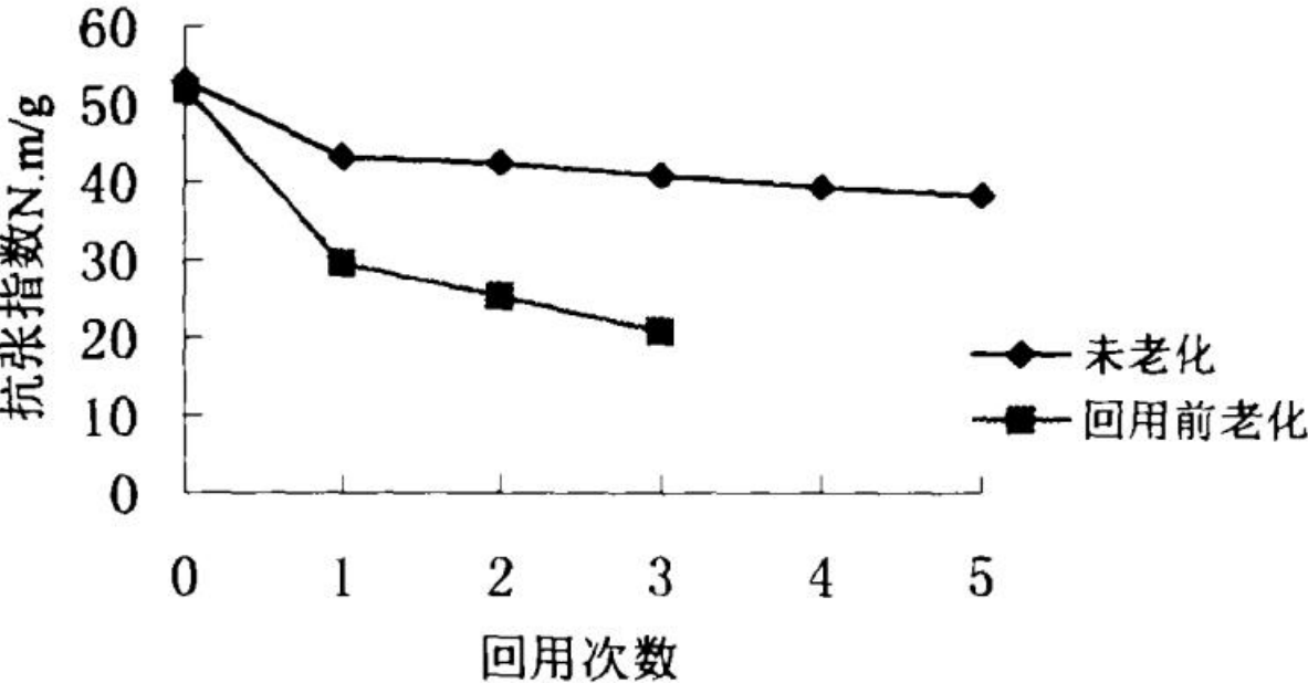
图5-10 回用过程中老化损伤变化
