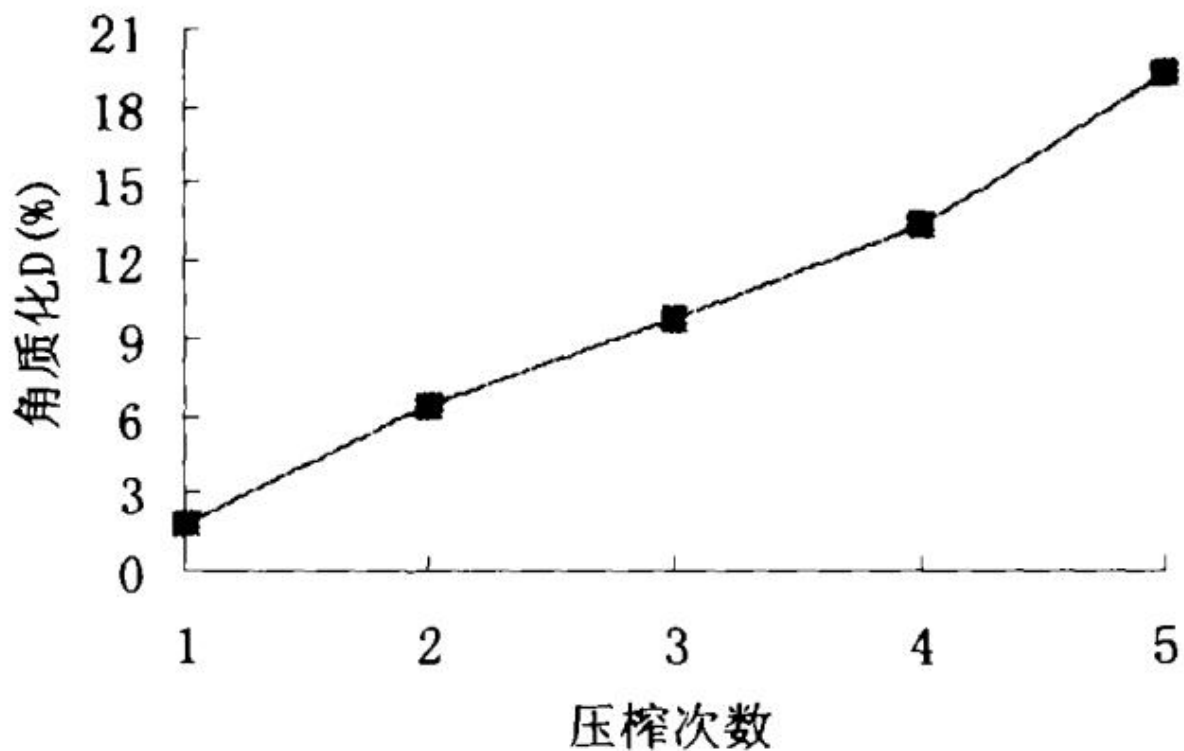
图3-9纤维角质化与压榨次数的关系
