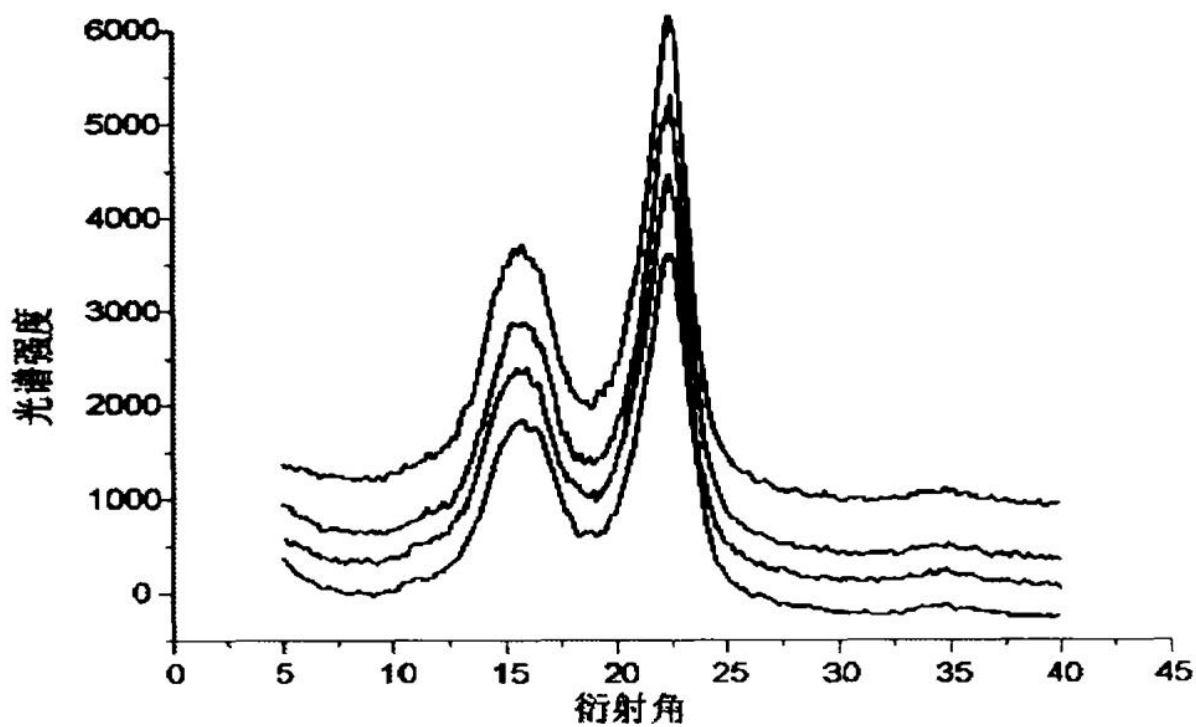
图2-3-1苇浆 X 一射线衍射图
