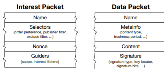
Figura 3: Pacotes das redes NDN [8]
