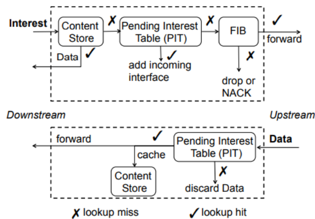
Figura 4: Processo de encaminhamento num nó NDN [8]
