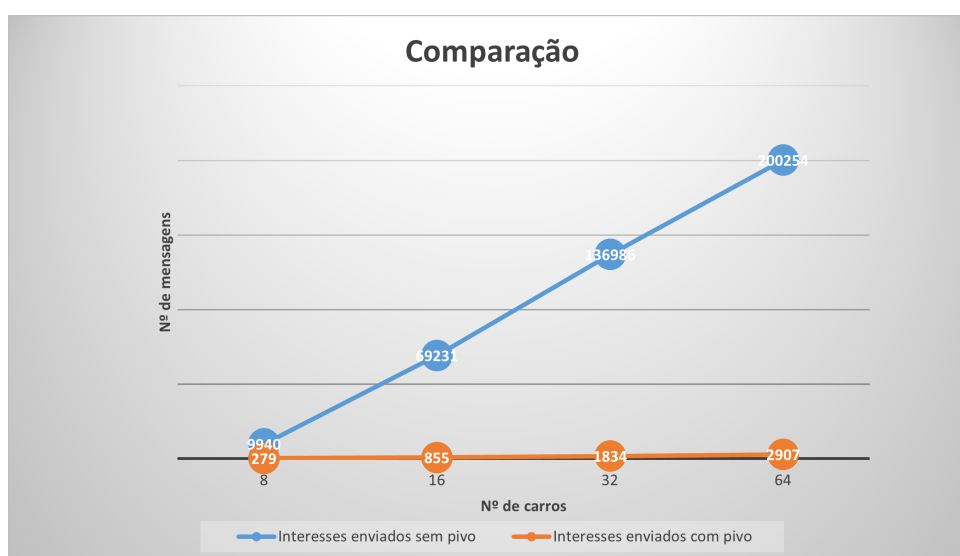
Figura 16: Evolução do número de interesses enviados com e sem pivô em função do número de carros.
