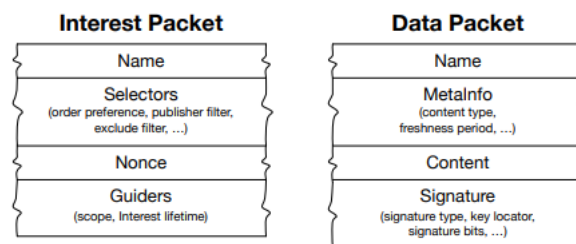
Figura 3: Pacotes das redes NDN [6]
