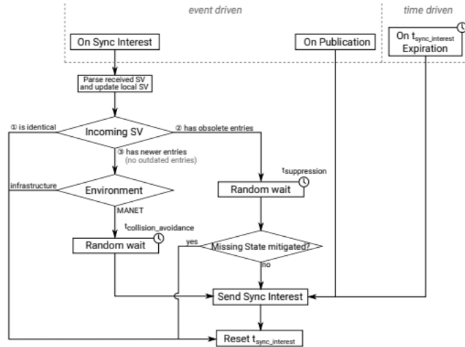
Figura 7: Fluxograma do funcionamento do SVSync [5]
