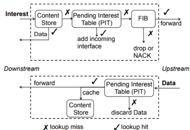
Figura 4: Processo de encaminhamento num nó NDN [6]
