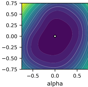
SGD
