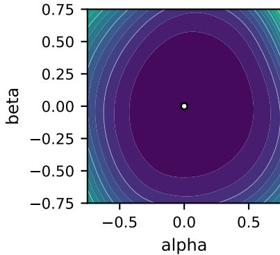
SAM
