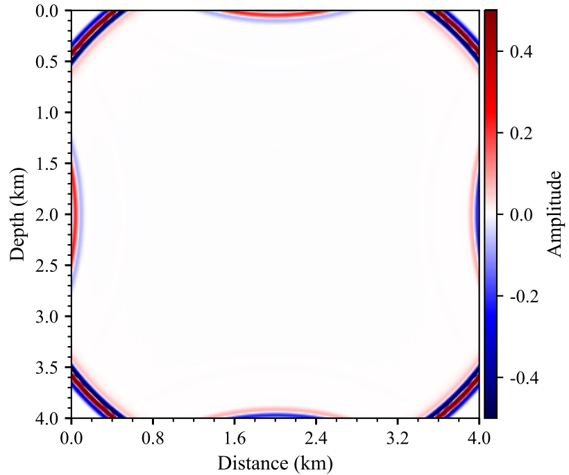
b. CPML边界条件
