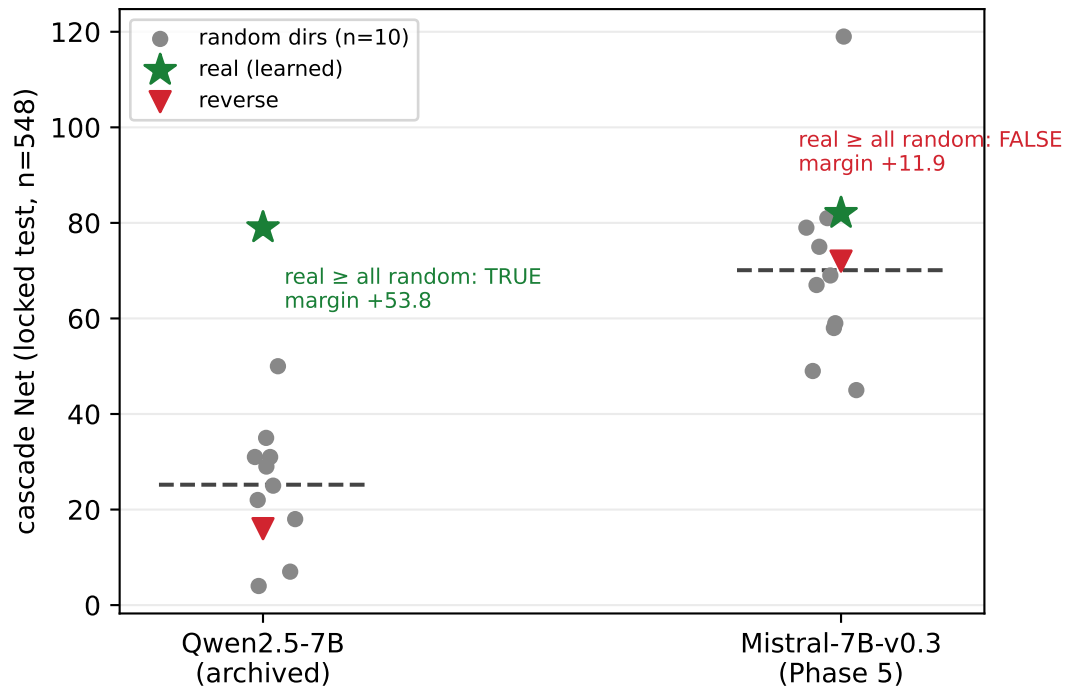
A. Cascade placebo: real vs random (same protocol, n_random=10)
