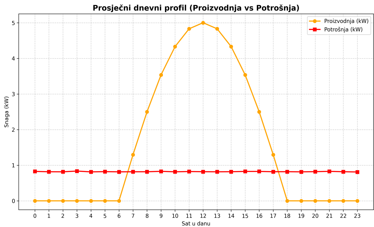
Slika 2: Prosječni dnevni profil proizvodnje i potrošnje.
