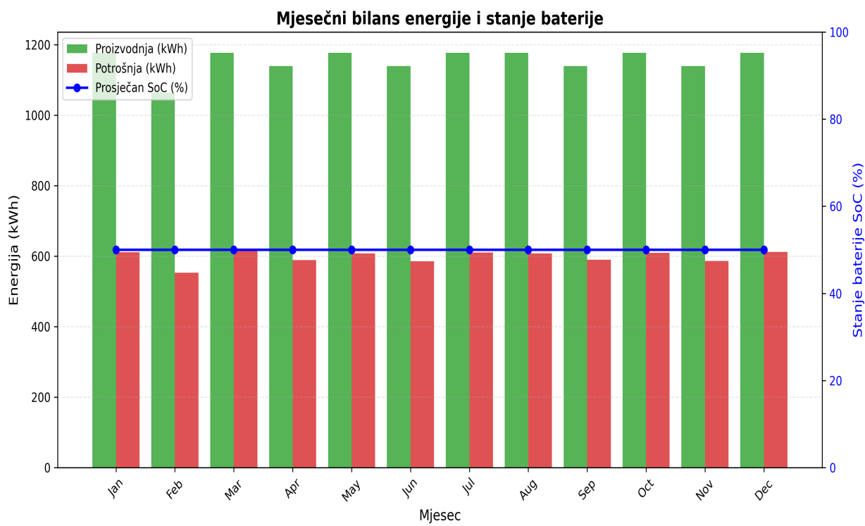
Slika 3: Mjesečni bilans energije i prosječno stanje baterije (SoC).
