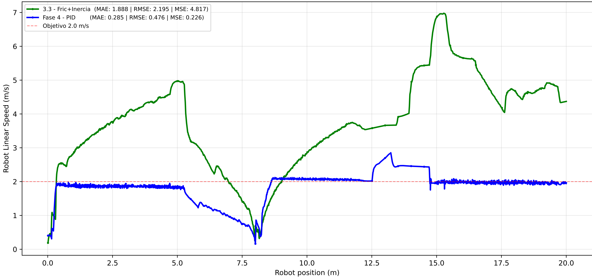
Fase 4 - Controlador PID vs Escenario 3.3
