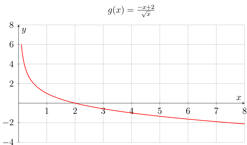
Figura 20. Gráfica de la función 2E g(x)
