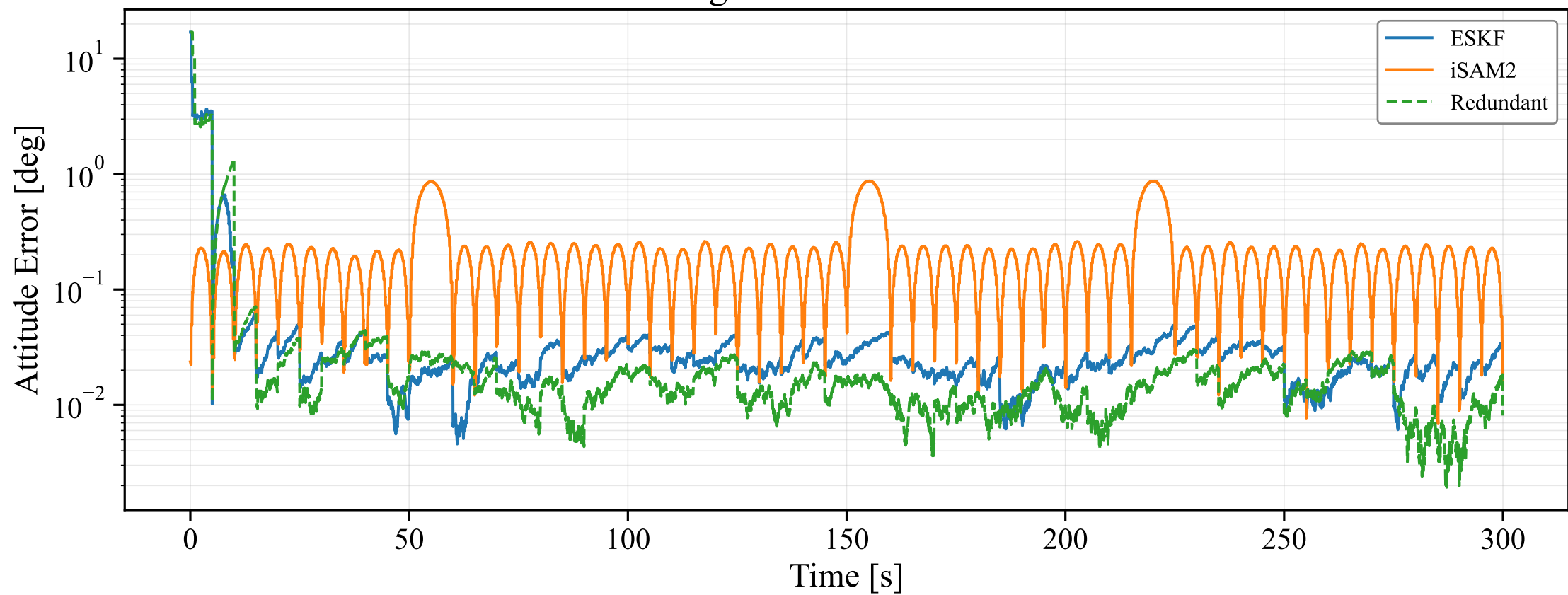
Mag Bias: Attitude Error
