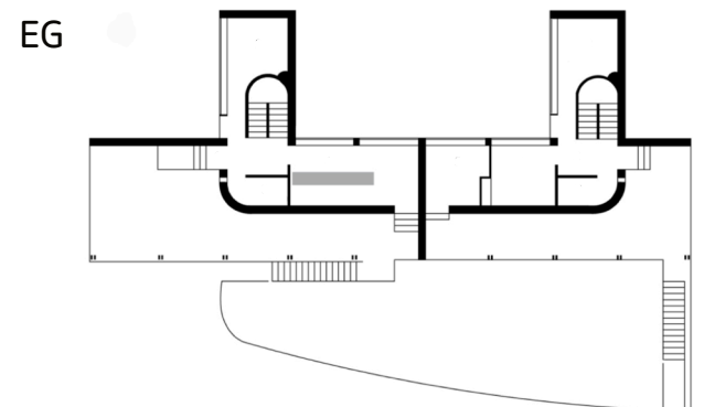
Grundrisse M 1:200
