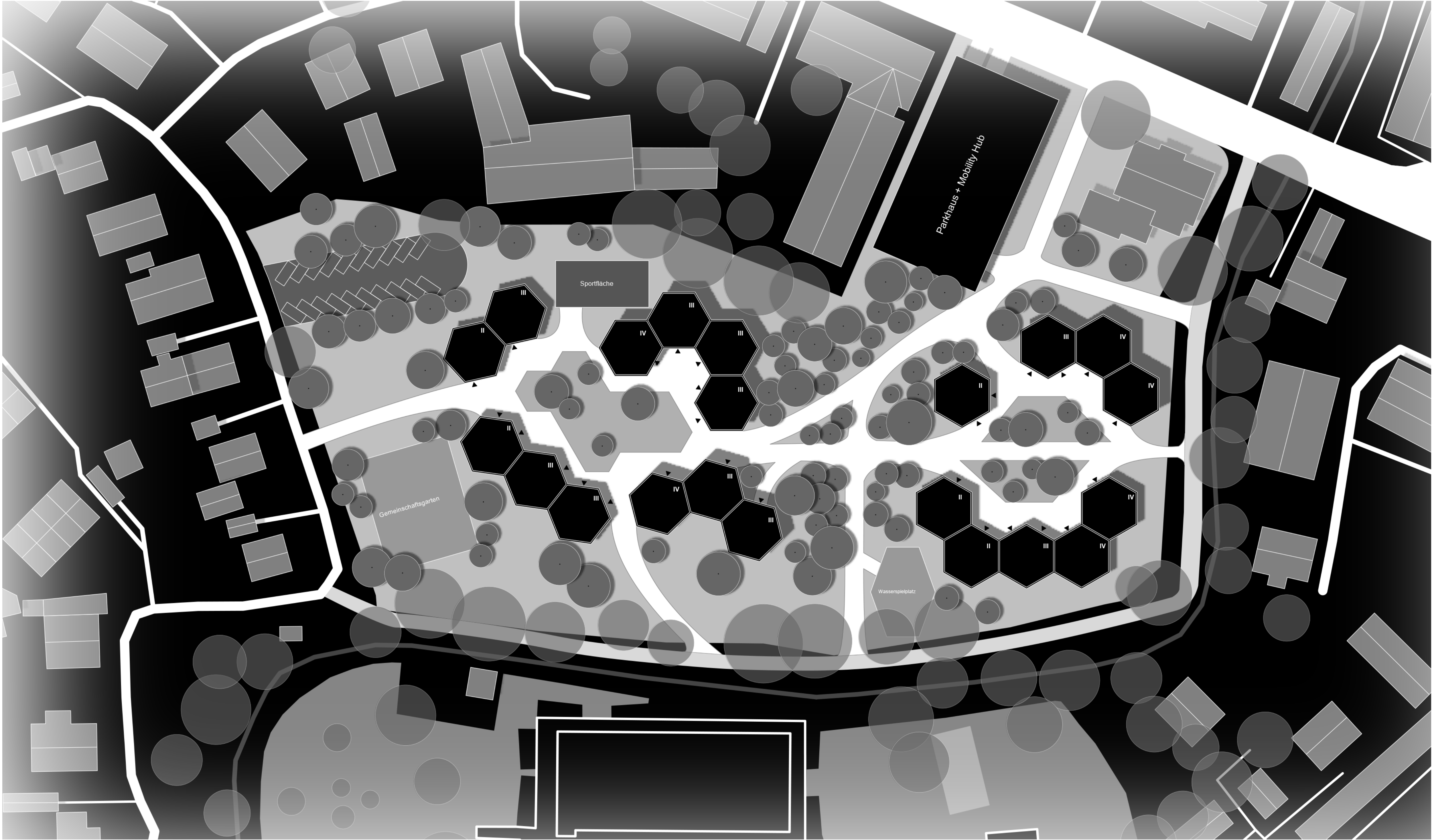
Lageplan 1:1000
