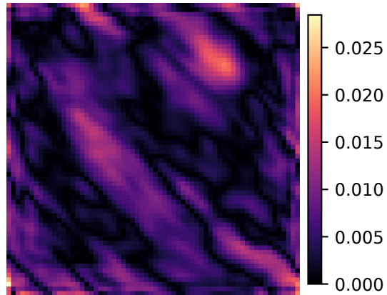
Absolute error
