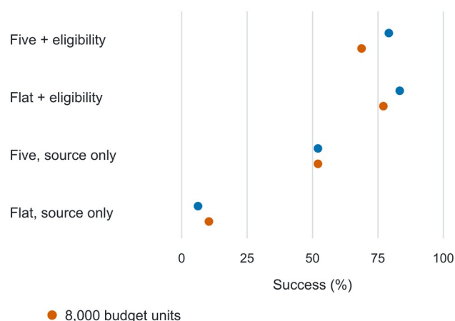
图3 完整操作一致性与反事实成对成功。点值直接由冻结聚合文件生成，分子和分母见表4；两预算分别使用96条相同轨迹和48对。未绘制不存在的独立重复运行误差棒。图示仅描述该合成样本与单个托管模型 alias。
