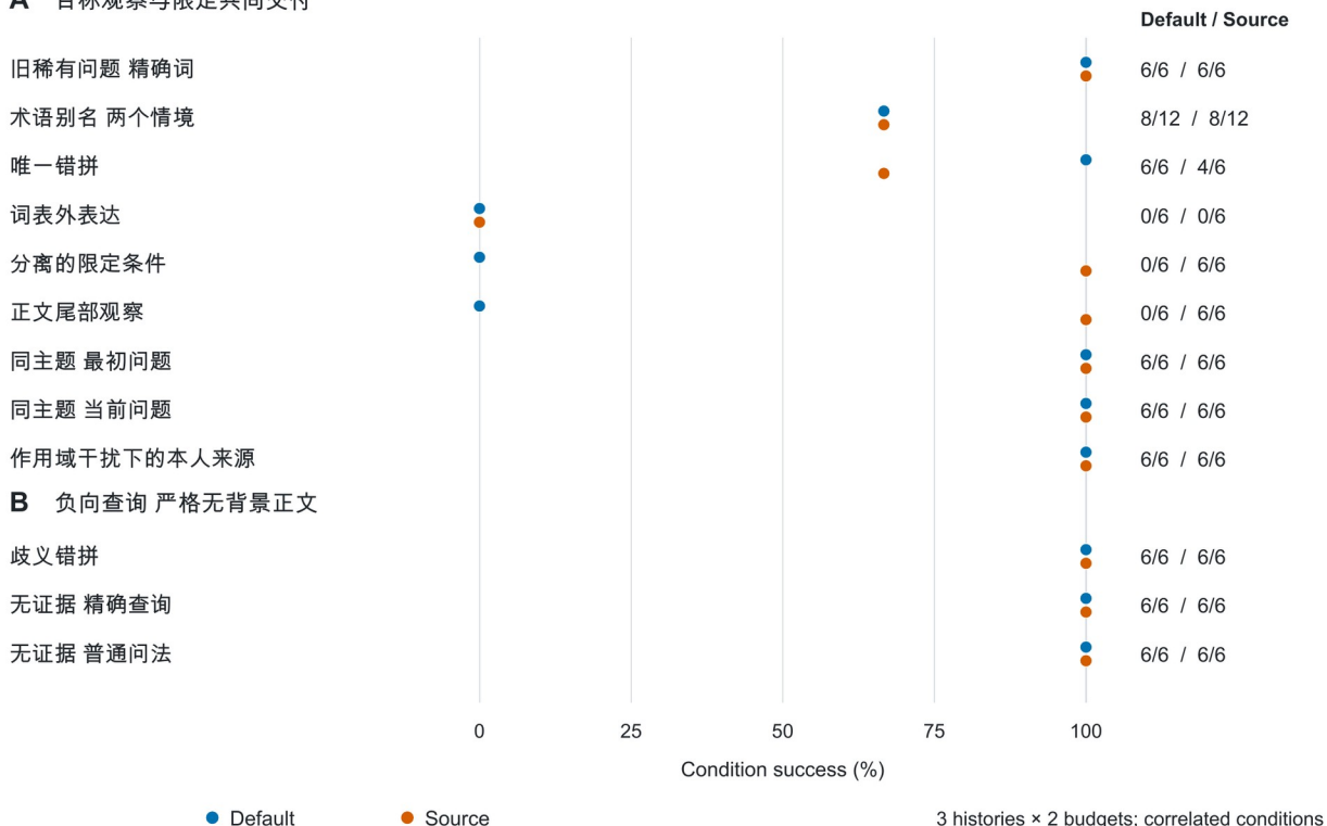
图5 默认与来源正文配置的分类型结果。A 为同条 Fact 中的目标观察与限定共同交付；B 为负向查询未携带有效背景正文。每个单情境含三档历史长度与两档预算，共 6 个相关条件；别名合并两个情境为 12 个条件。右侧明确给出默认/原文配置分子分母，未构造独立重复或总体置信区间。局部开关消融结果另列补充材料，不混入共同配置分母。
