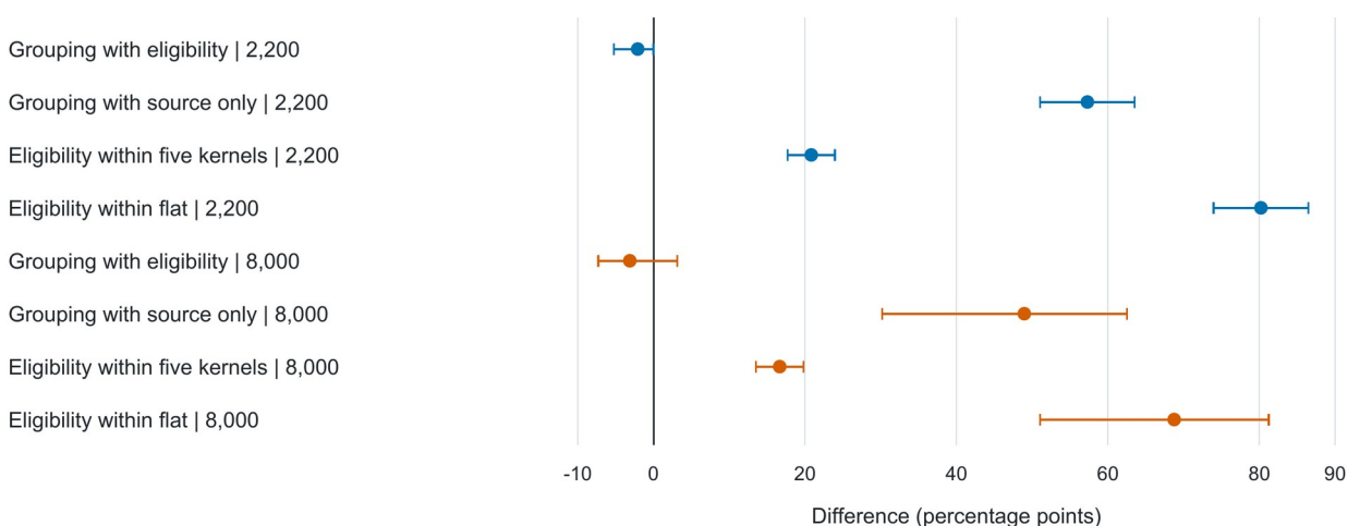
图4 完整操作一致性的配对差异。Grouping 表示五核减平面，Eligibility 表示加资格注释减仅来源。区间接八个作者生成主题簇计算，仅作探索性描述。横轴单位为百分点，分组的细小差异还受到下述输出契约影响。
