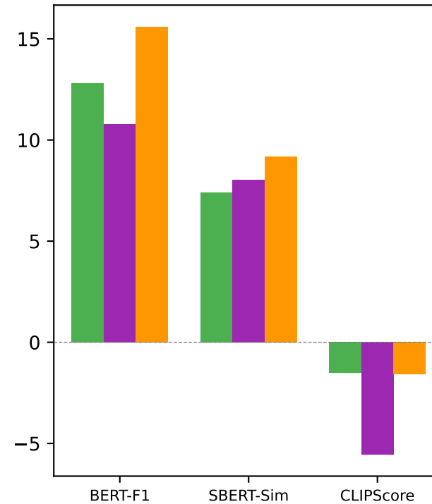
Gemma-3-27B
