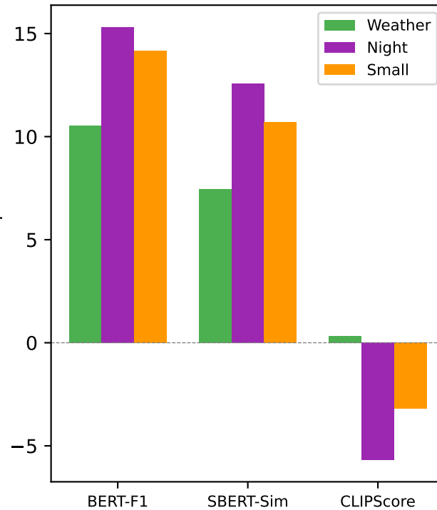
Phi-4
