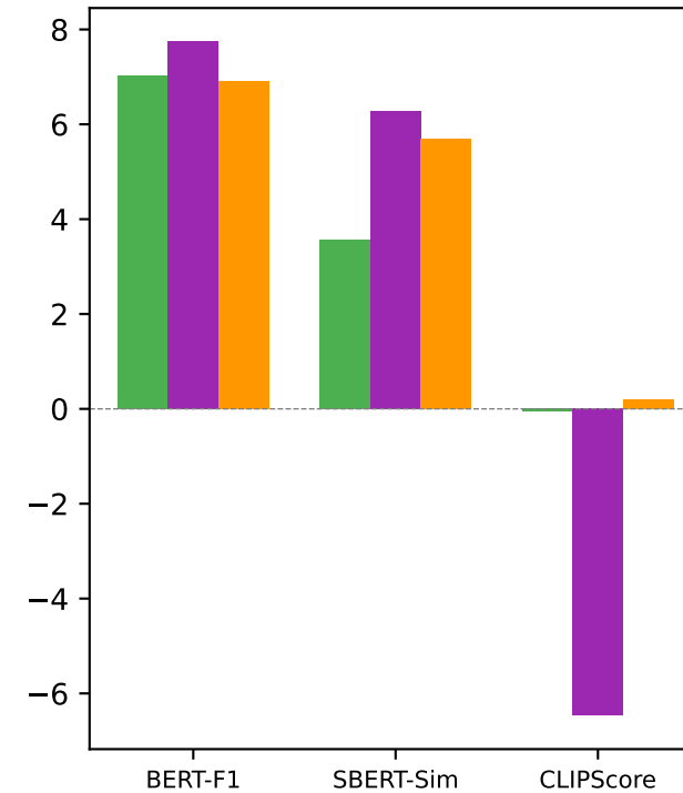
LLaVA-1.5-7B
