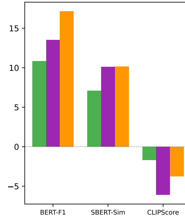
Qwen3-VL-8B
